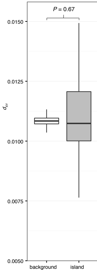
C.pauper_F vs. L.noctis
