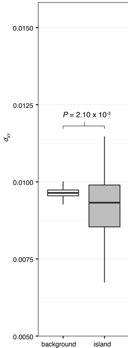
G.magnirostris_G vs. L.noctis
