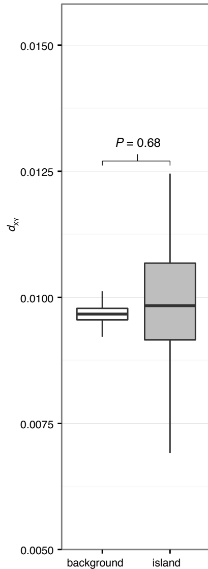
P.inornata_C vs. L.noctis
