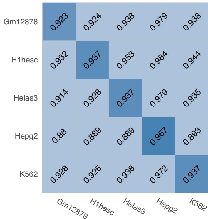
NRF1 (Interaction)
