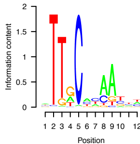
CEBPB-M00912
