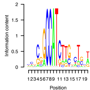
YY1-M00069
