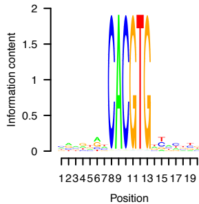
MYC-M00615
