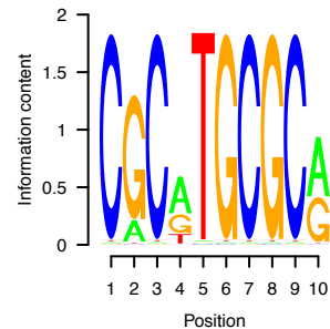
NRF1-M00652
