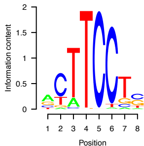
GABPA-M00971
