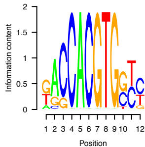
MYC-M01154
