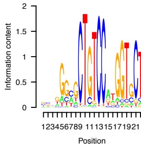
REST-M01256
