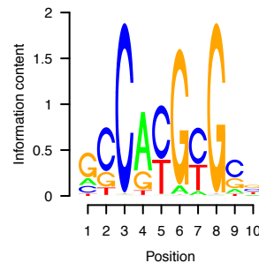
MYC-M00322
