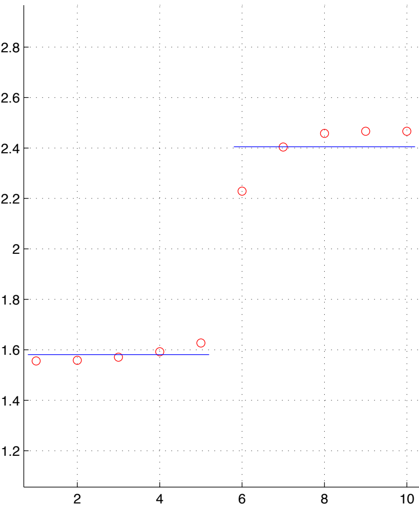
LUAD-3-T.chainID.2 numStates=2
