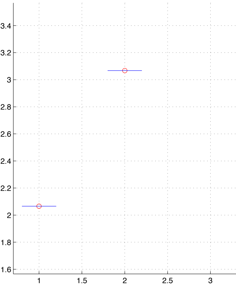
OV-3-T.chainID.5 numStates=2
