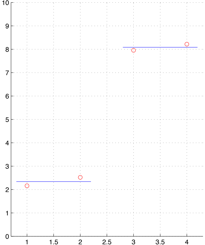
LUSC-3-T.chainID.2 numStates=2
