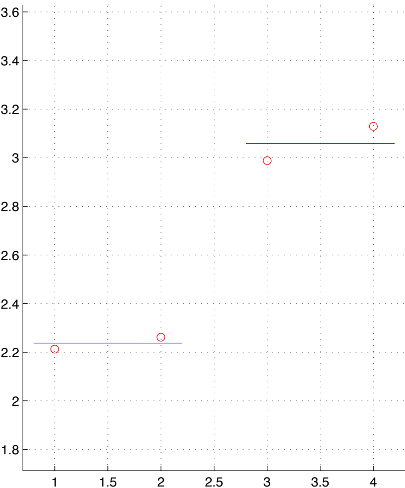
OV-6-T.chainID.2 numStates=2
