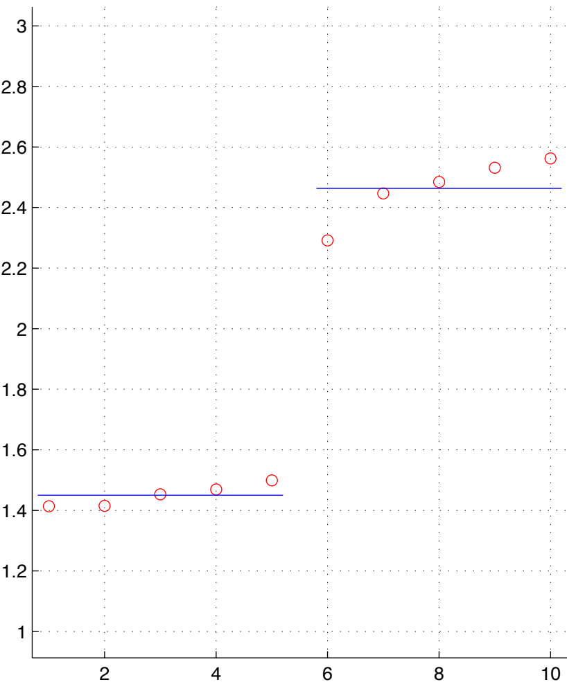
OV-7-T.chainID.1 numStates=2
