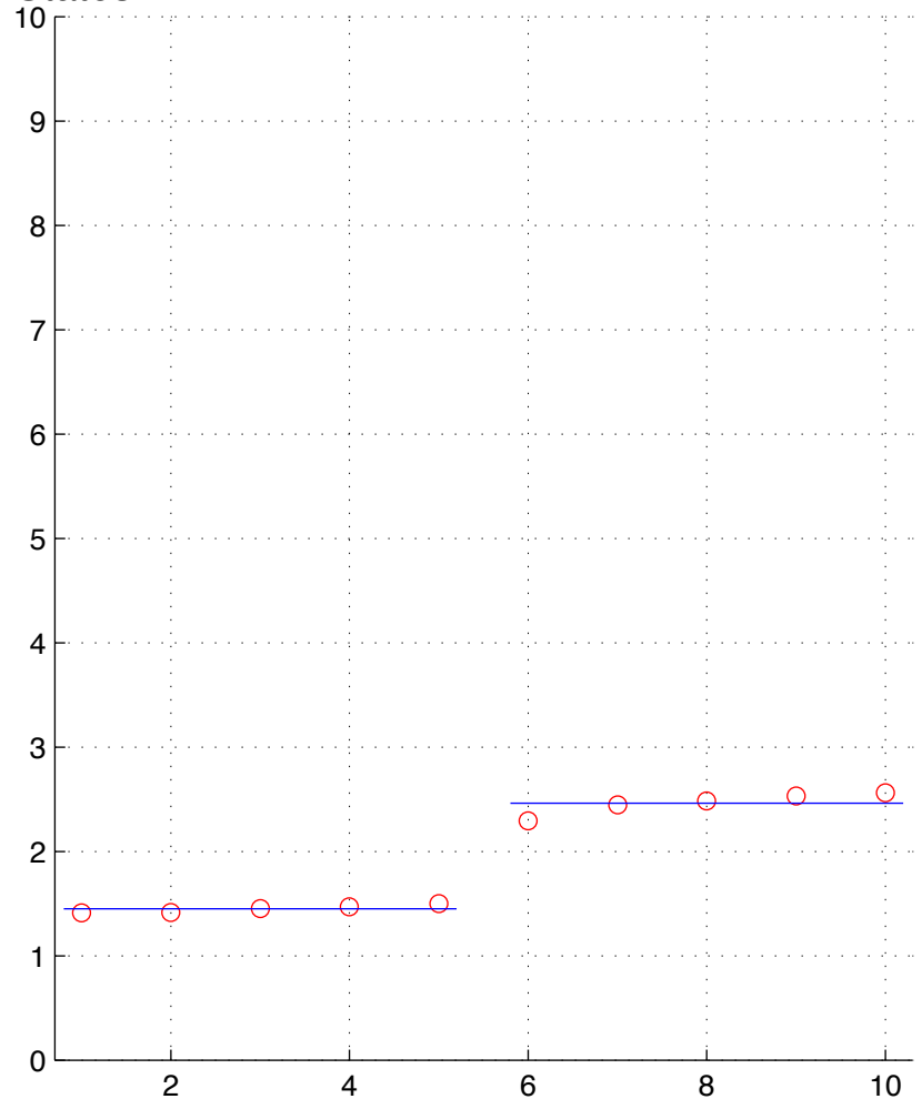
OV-7-T.chainID.1 numStates=2
