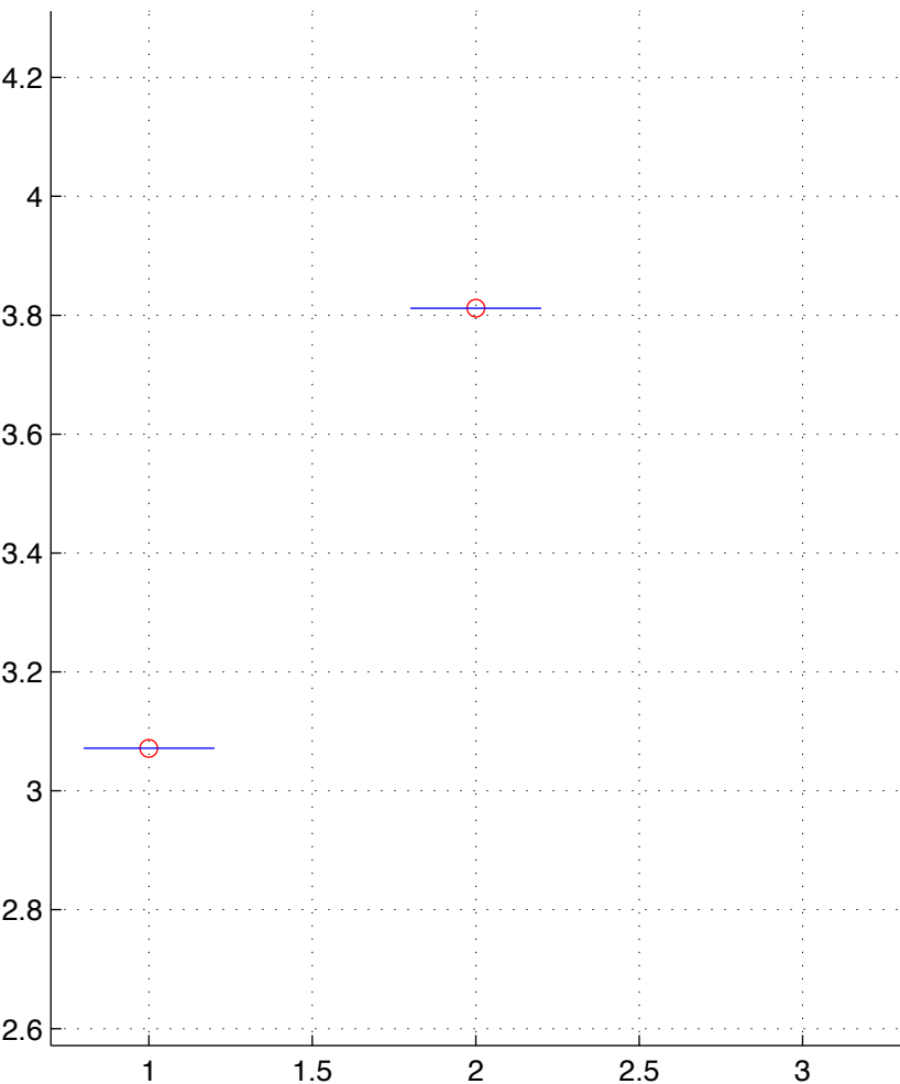
OV-1-T.chainID.3 numStates=2
