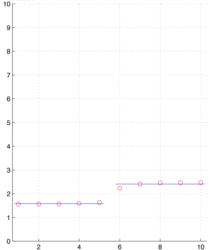
LUAD-3-T.chainID.2 numStates=2
