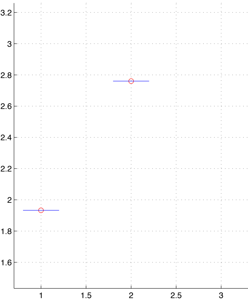
OV-3-T.chainID.1 numStates=2
