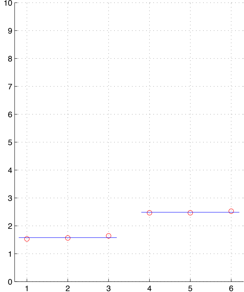
LUAD-3-T.chainID.3 numStates=2
