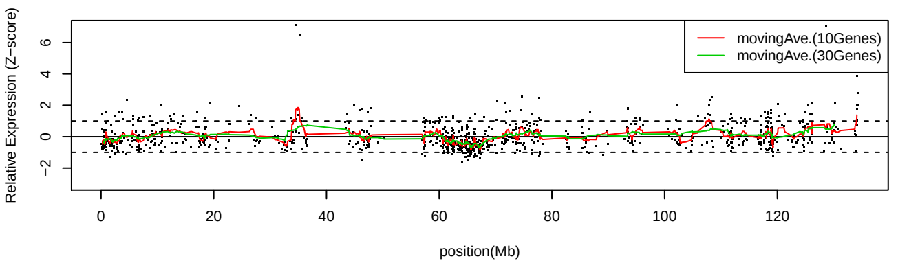
LC_S5 Chr11
