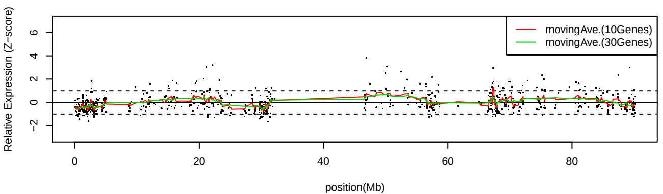
LC_S5 Chr16
