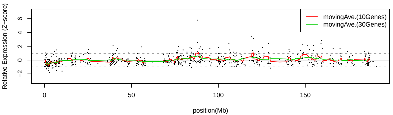
LC_S5 Chr4
