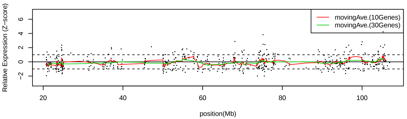
LC_S51 Chr14
