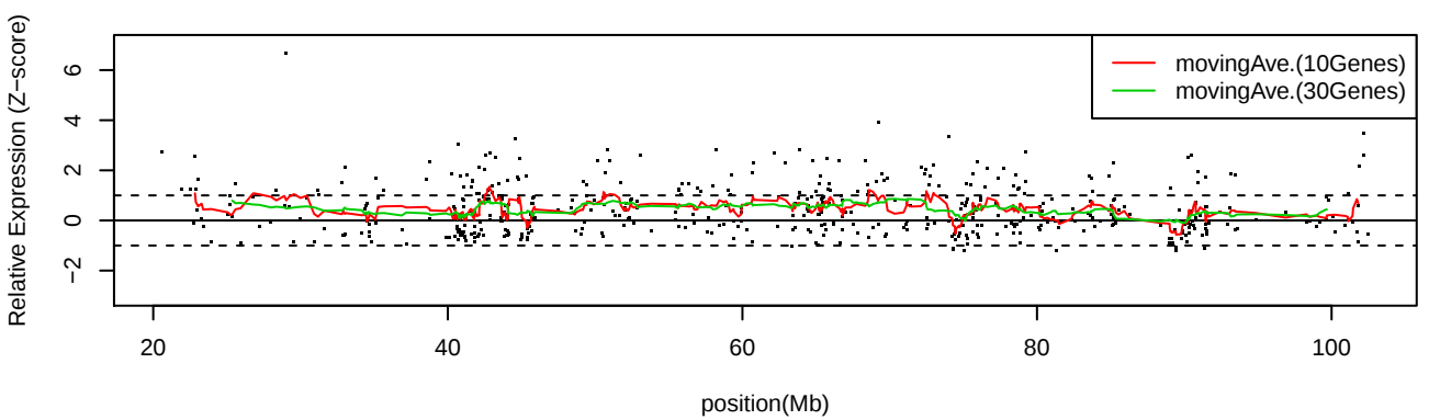
LC_S5 Chr15
