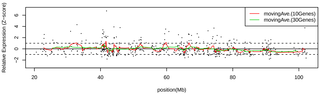
LC_S4 Chr15
