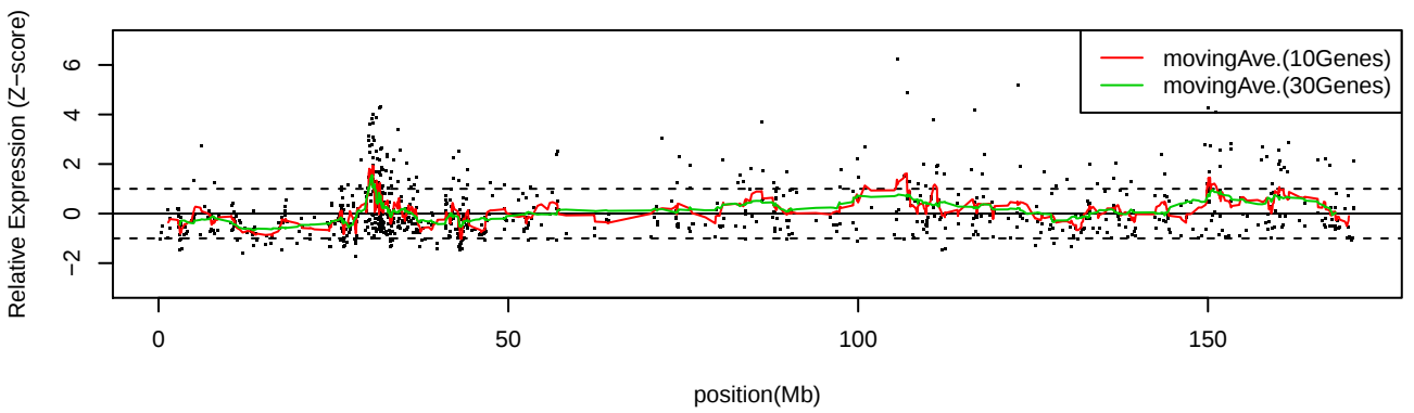
LC_S4 Chr6
