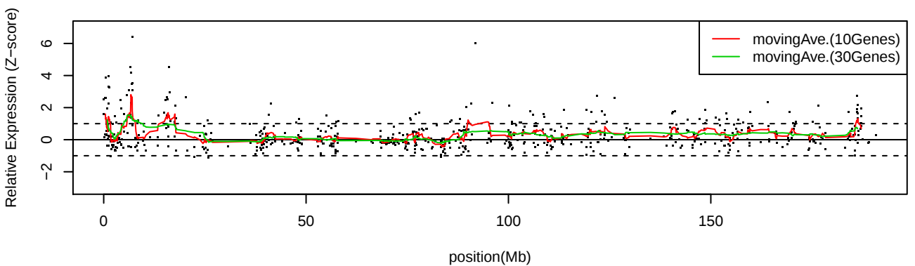
LC_S50 Chr4
