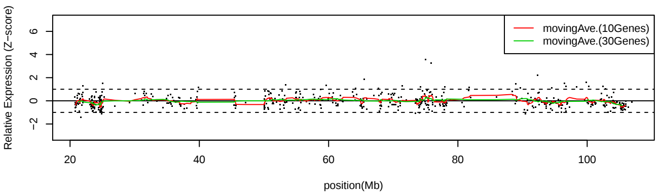
LC_S50 Chr14
