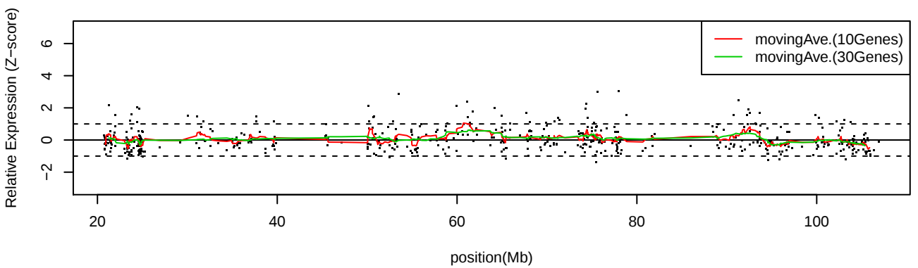
LC_S5 Chr14
