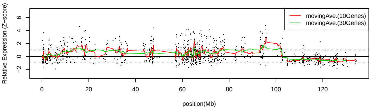
LC_S3 Chr11
