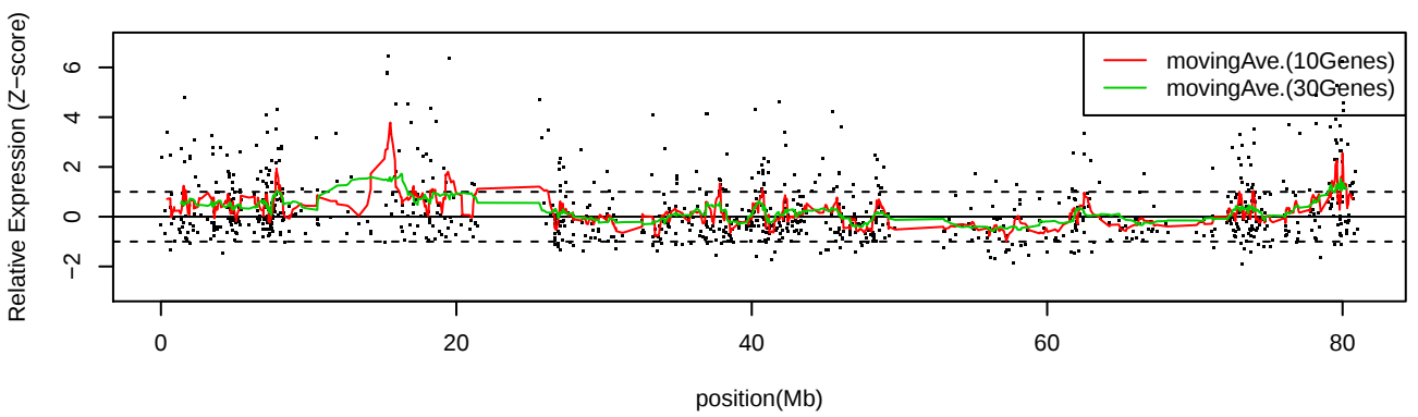
LC_S27 Chr17
