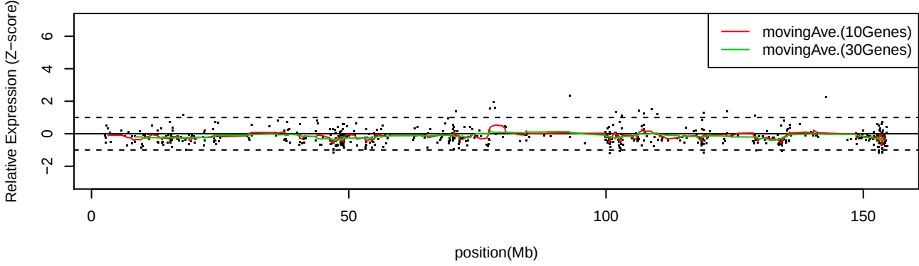
LC_S28 ChrX
