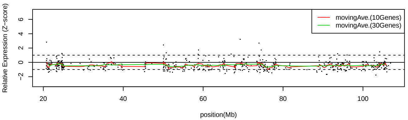
LC_S21 Chr14
