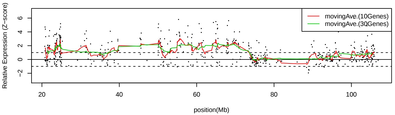
LC_S25 Chr14
