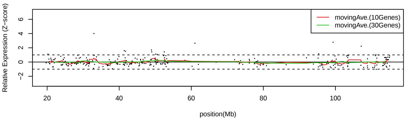
LC_S30 Chr13
