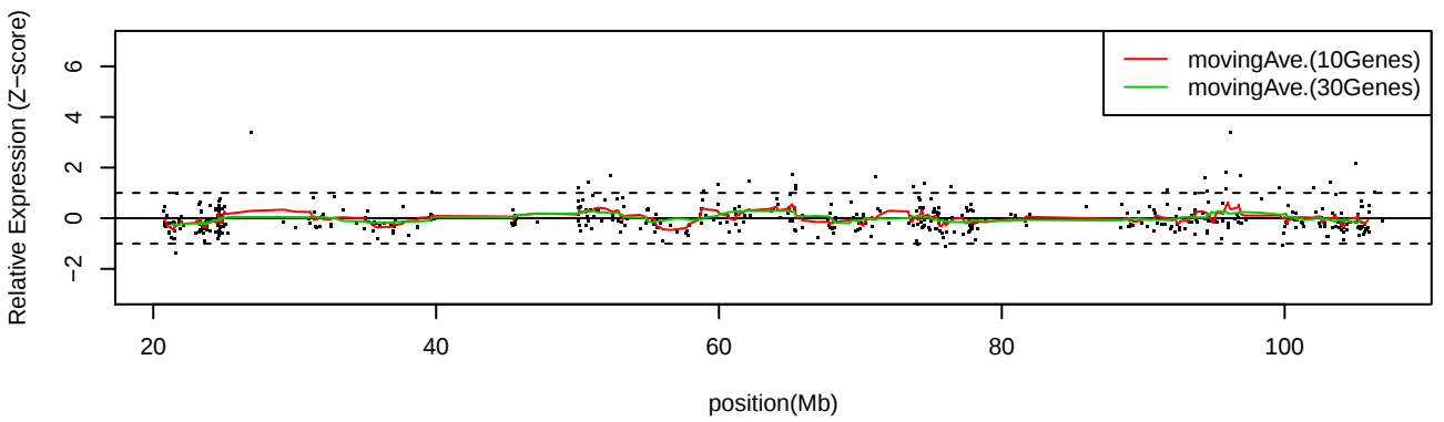
LC_S28 Chr14
