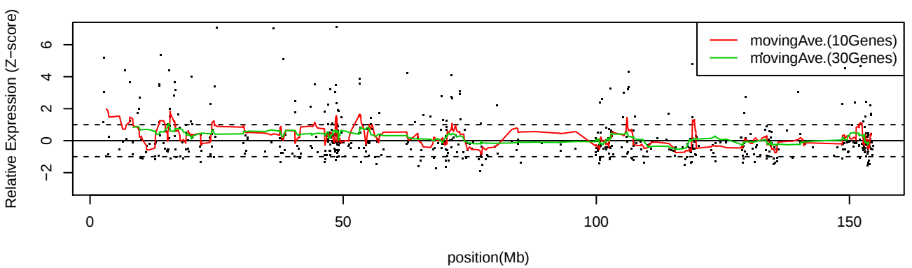
LC_S23 ChrX
