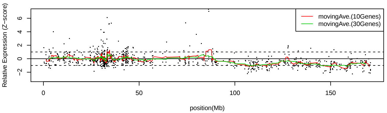
LC_S21 Chr6
