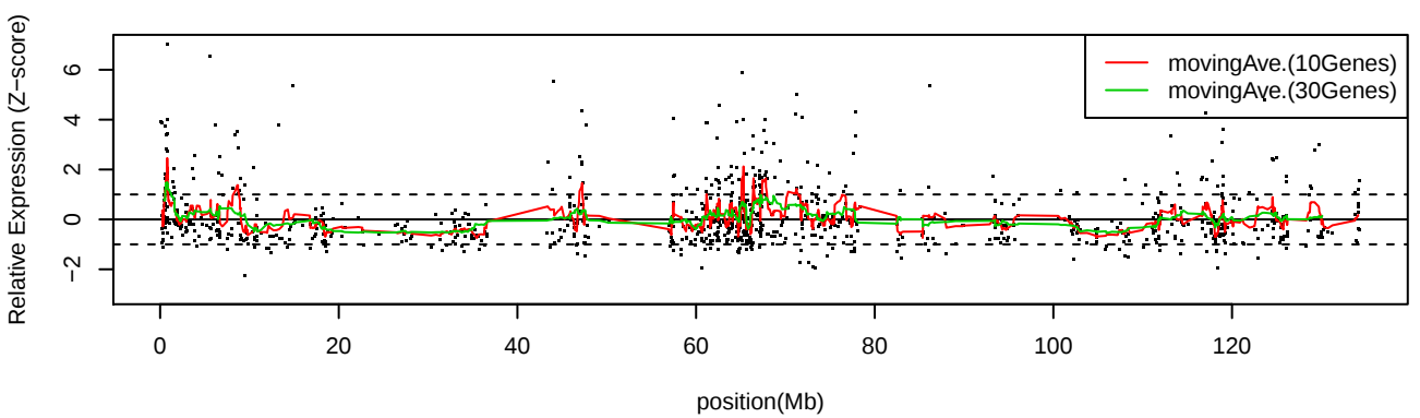
LC_S27 Chr11
