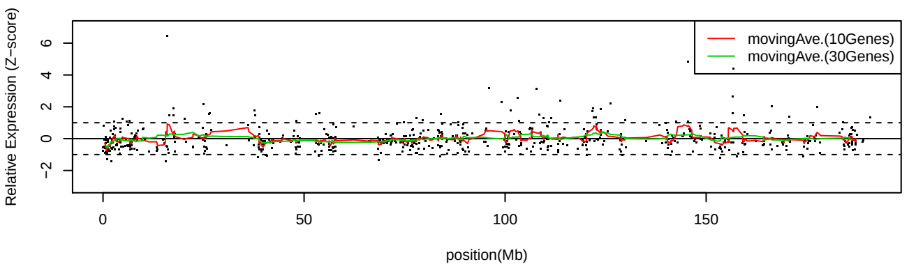
LC_S22 Chr4
