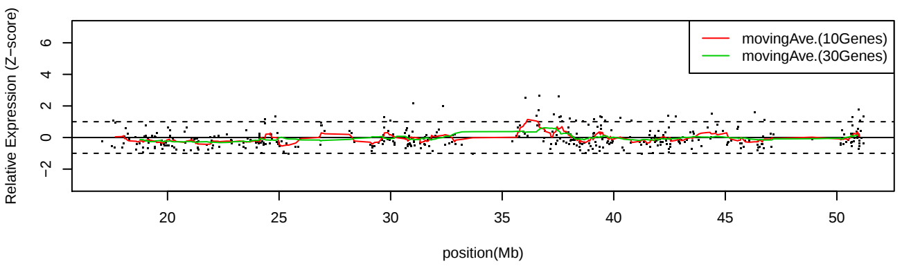
LC_C32 Chr22
