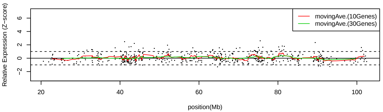
LC_C35 Chr15
