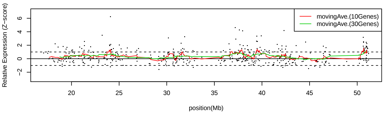
LC_S8 Chr22
