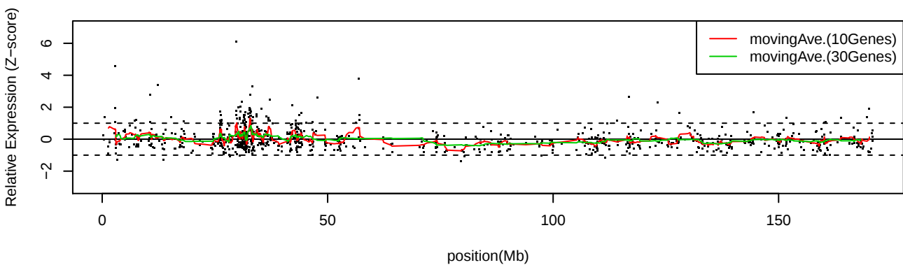
LC_C32 Chr6
