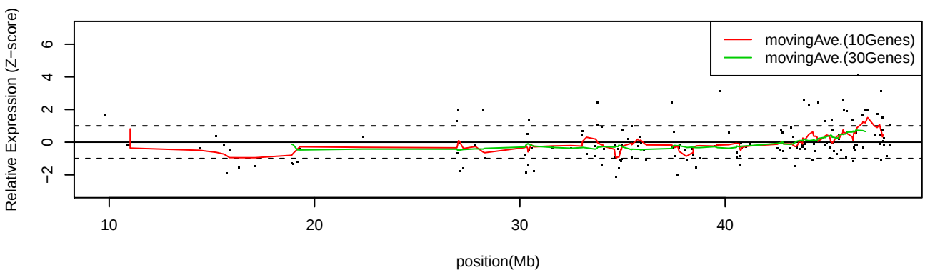
LC_S6 Chr21
