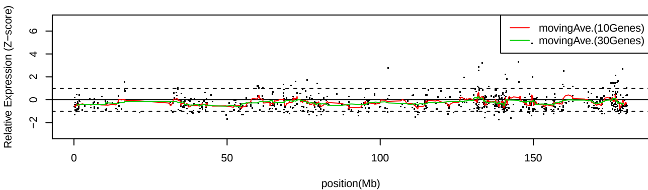
LC_C33 Chr5
