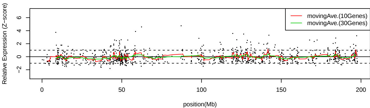
LC_C33 Chr3
