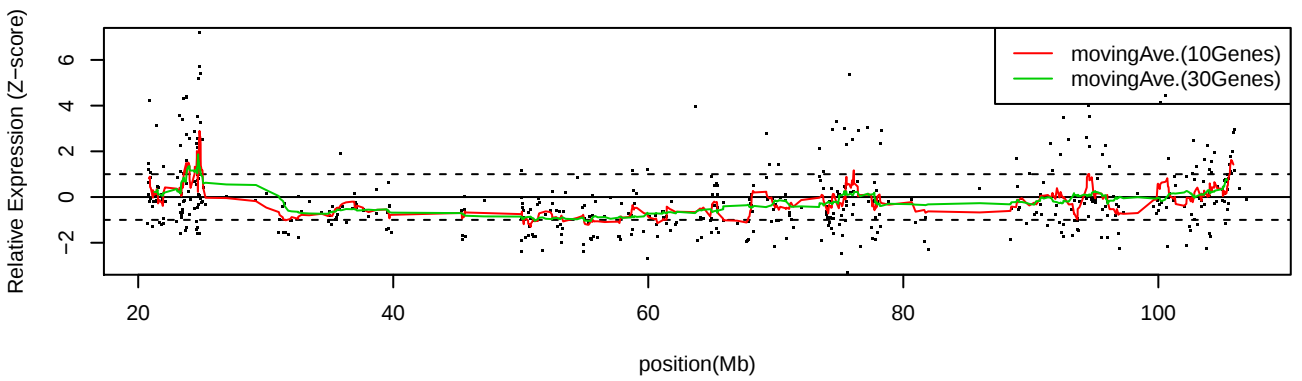
LC_S6 Chr14
