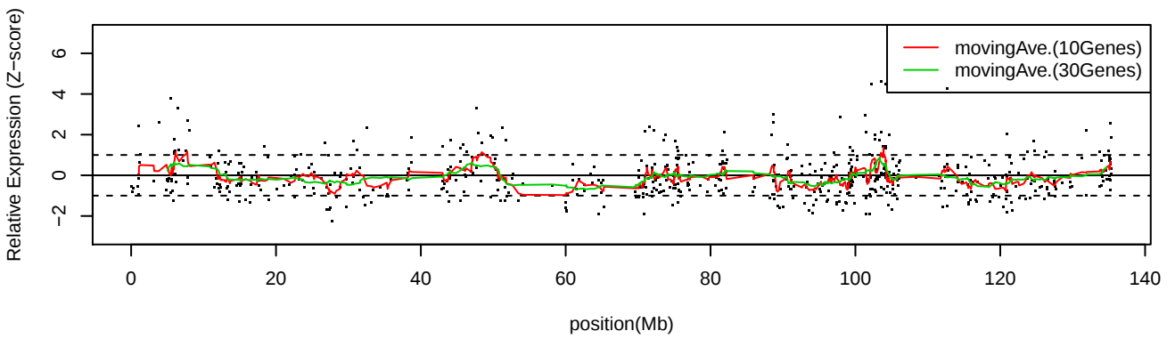
LC_S8 Chr10
