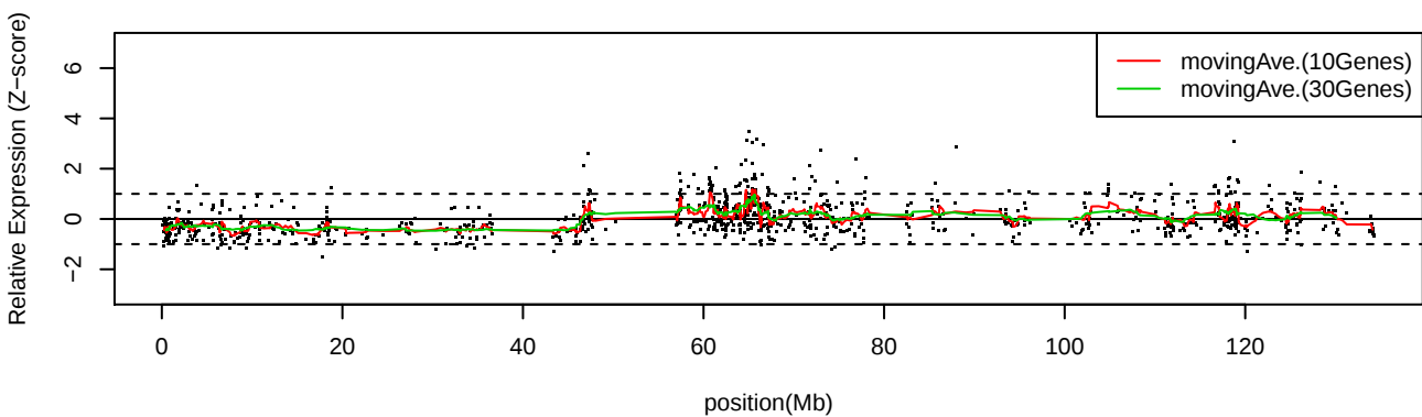
LC_C32 Chr11
