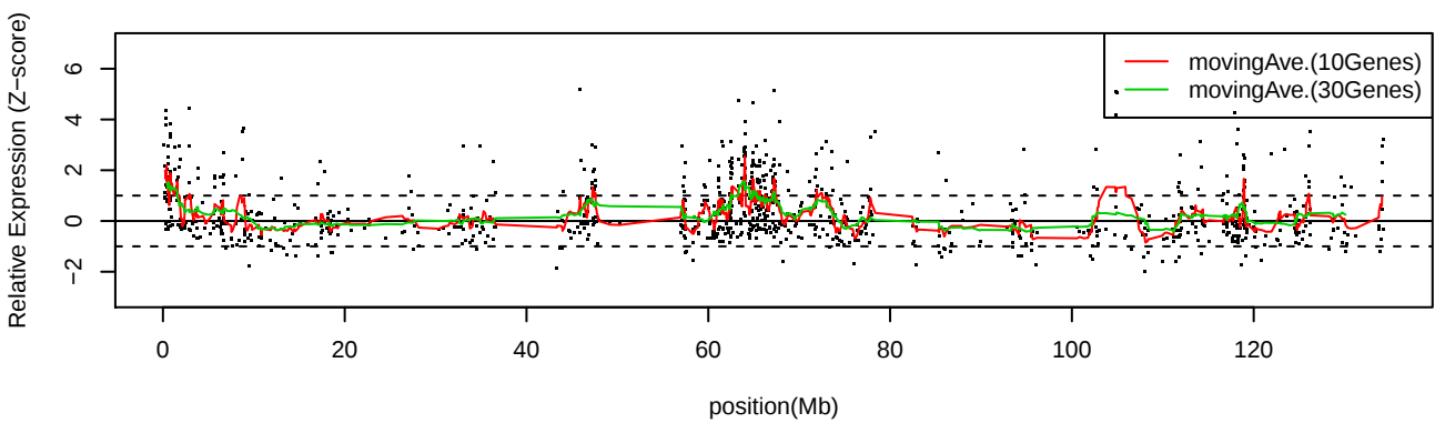
LC_S9 Chr11
