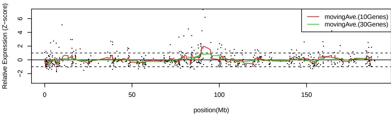
LC_C31 Chr4
