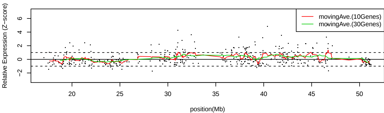
LC_C33 Chr22
