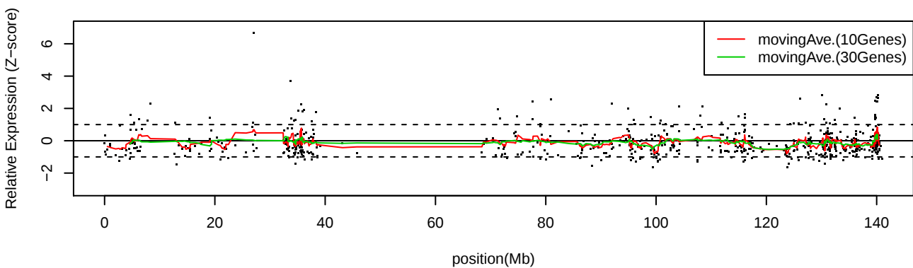
LC_C33 Chr9
