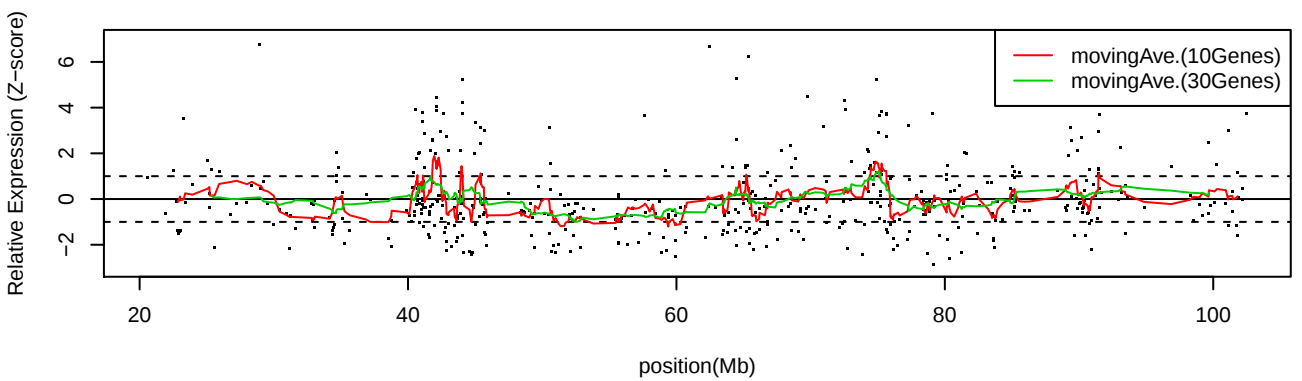
LC_S6 Chr15
