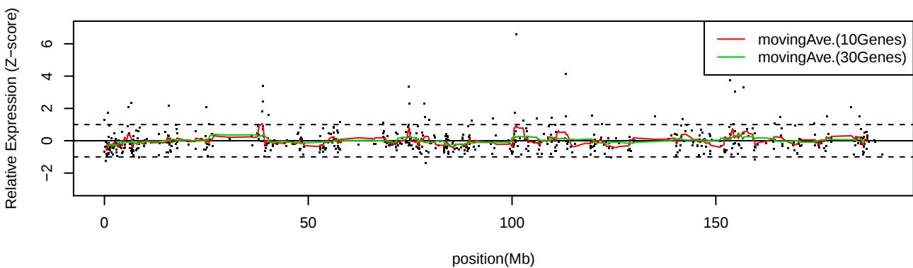
LC_C35 Chr4
