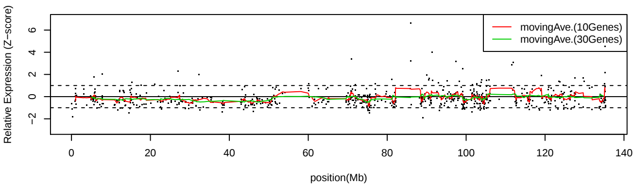
LC_C33 Chr10
