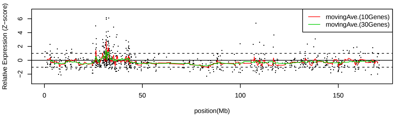
LC_S8 Chr6
