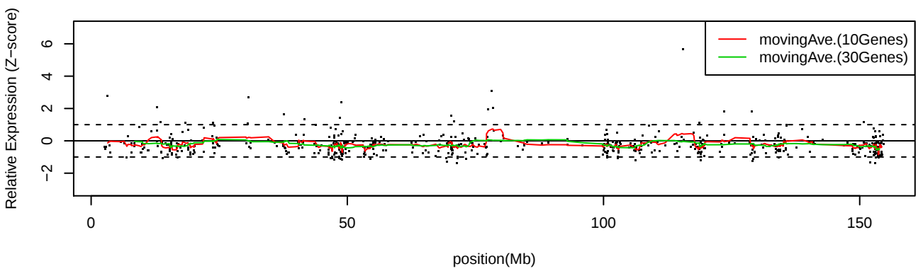
LC_C35 ChrX
