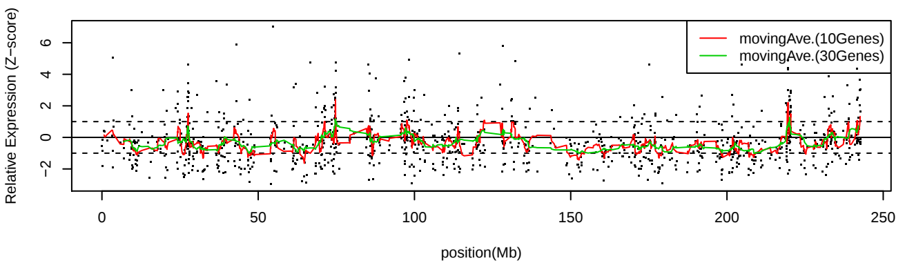
LC_S6 Chr2
