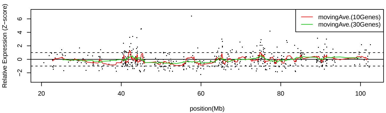
LC_S8 Chr15
