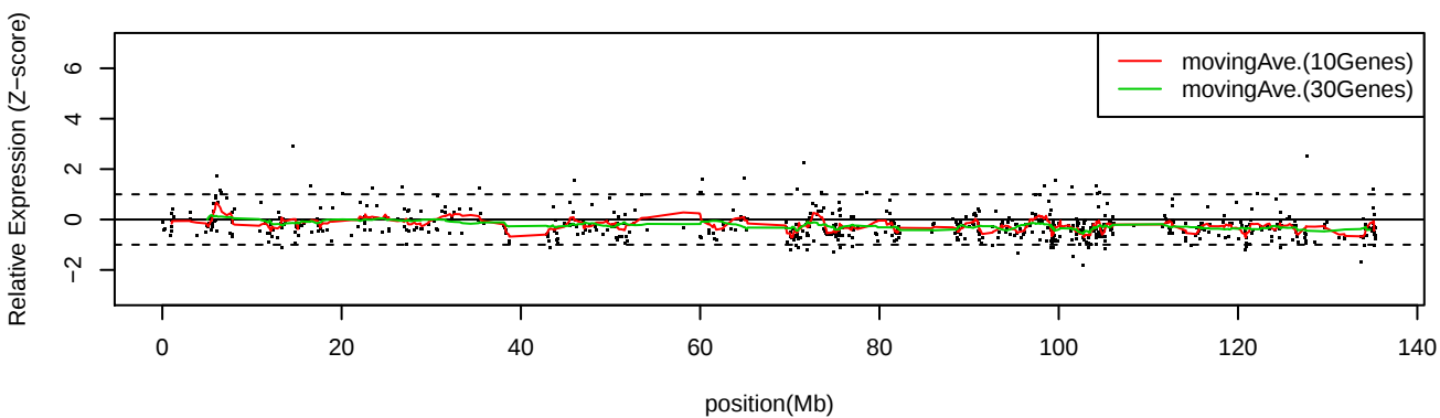
LC_C35 Chr10
