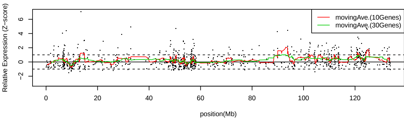
LC_C33 Chr12
