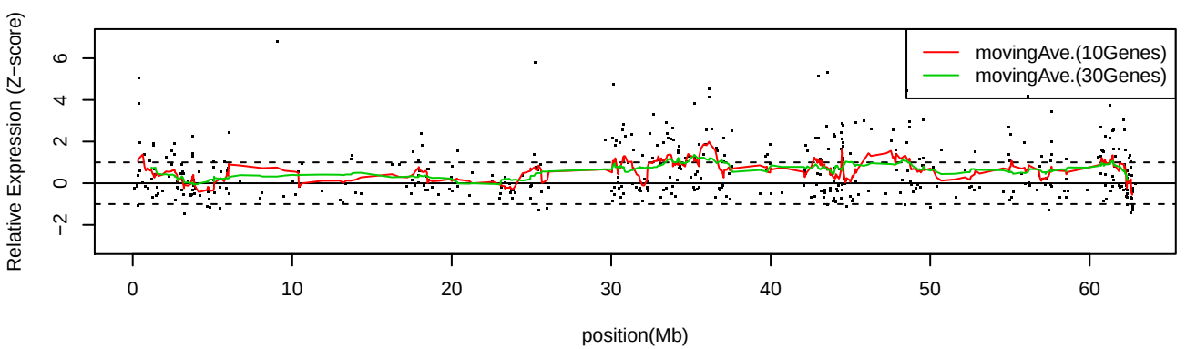
LC_C33 Chr20
