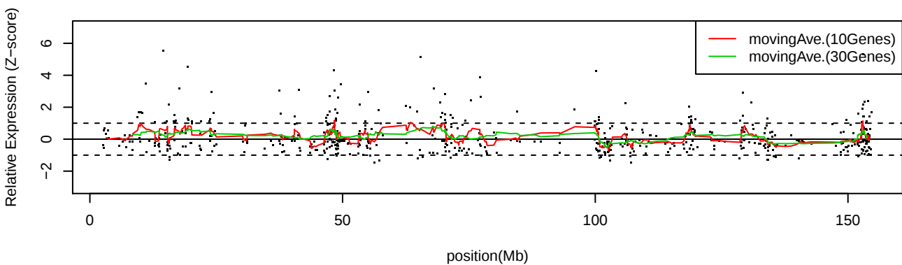
LC_C33 ChrX
