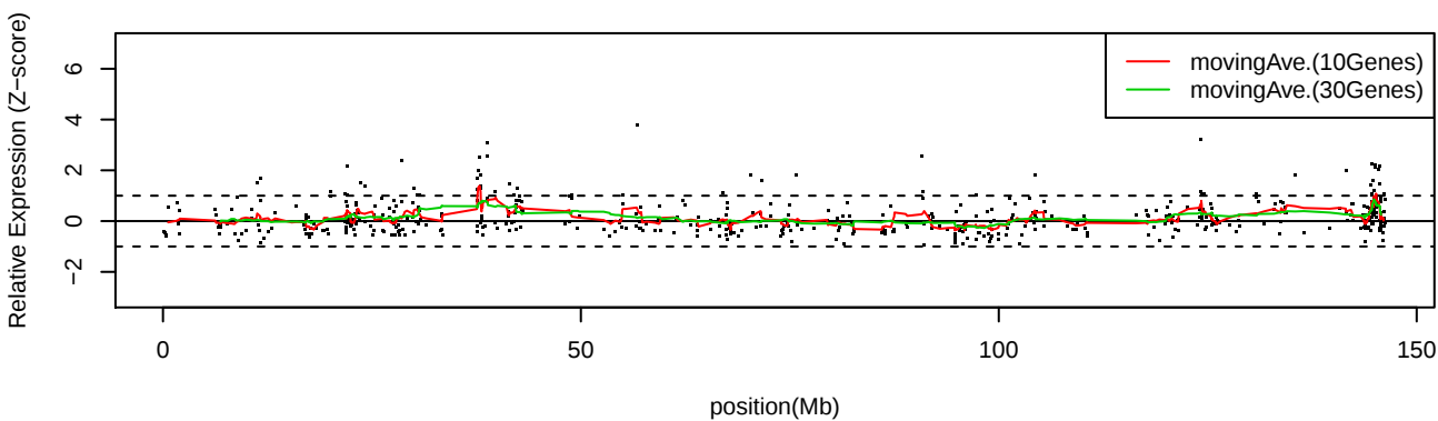
LC_C32 Chr8
