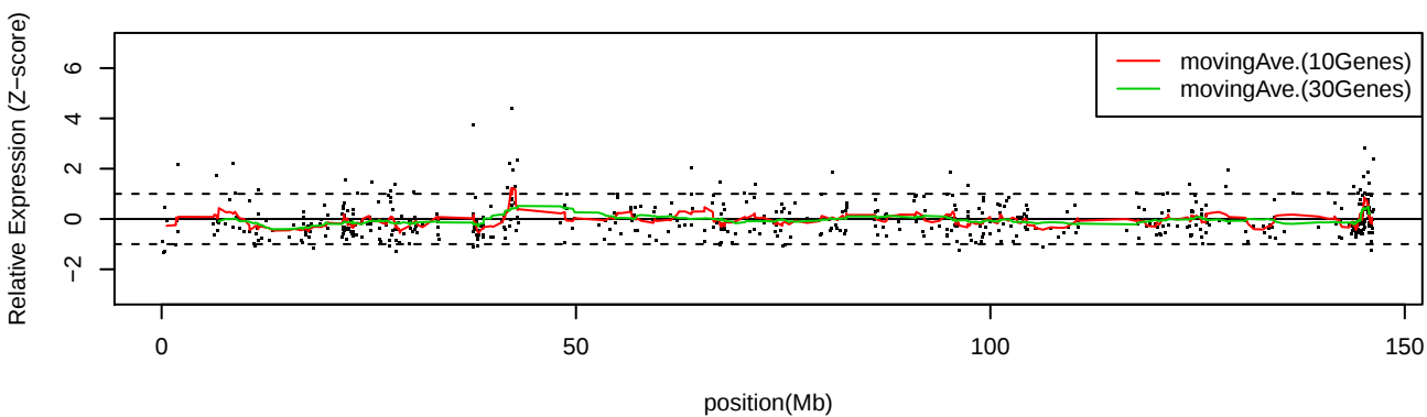
LC_C33 Chr8
