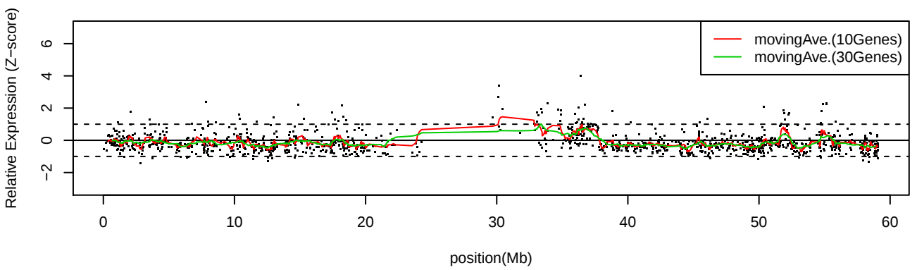
LC_C32 Chr19
