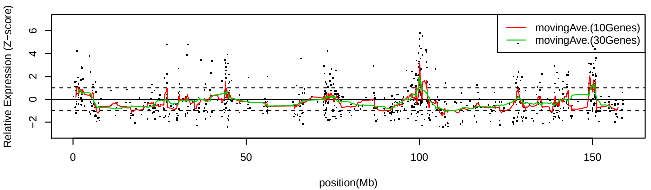
LC_S6 Chr7
