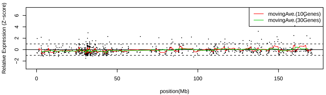
LC_C35 Chr6
