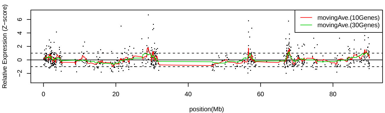
LC_S8 Chr16
