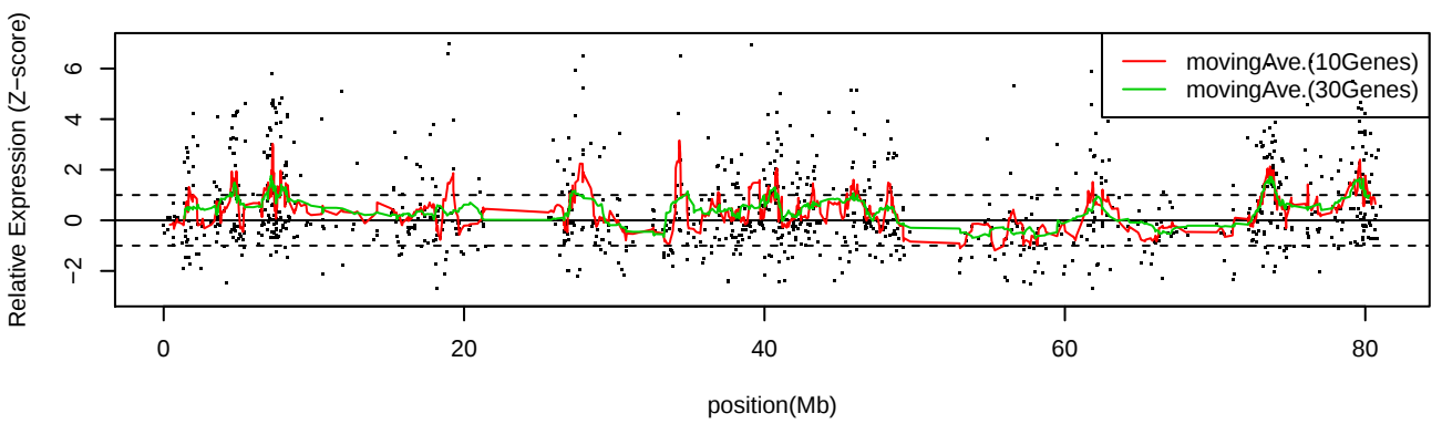
LC_S6 Chr17
