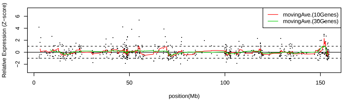
LC_C34 ChrX
