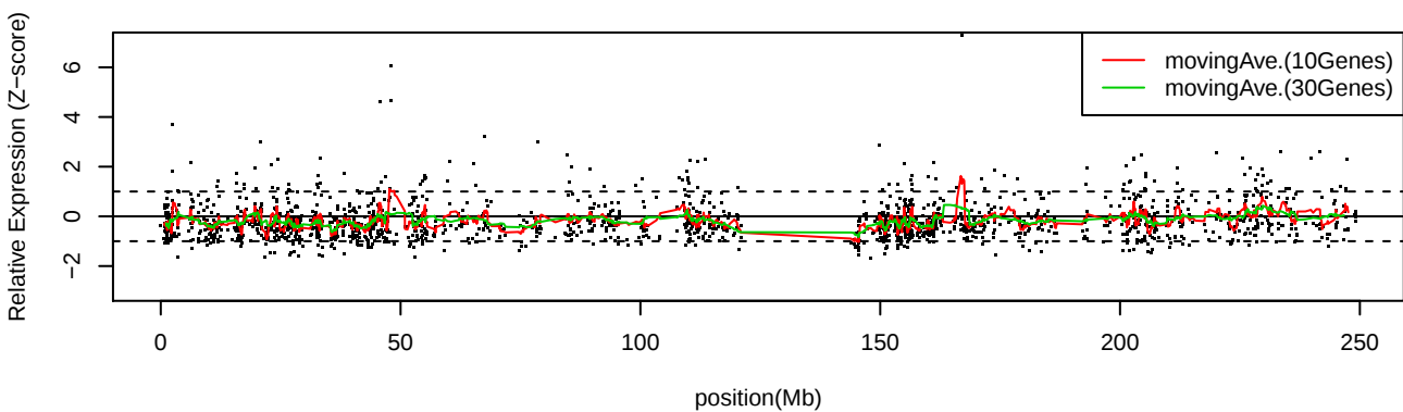
LC_C33 Chr1
