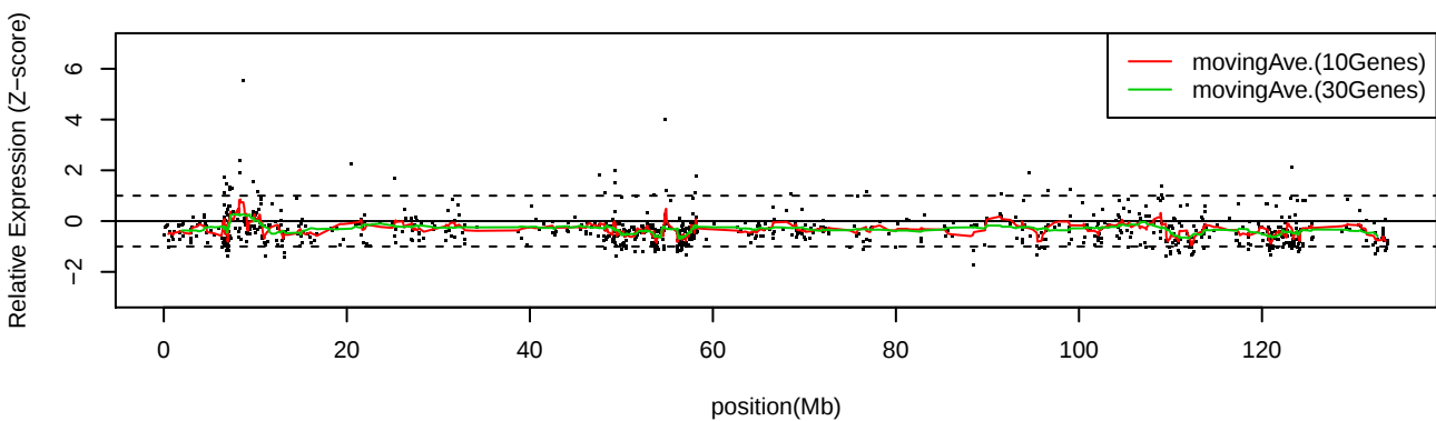
LC_C35 Chr12
