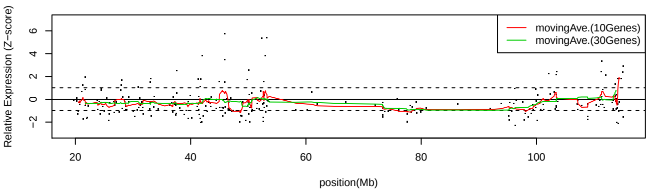
LC_S6 Chr13
