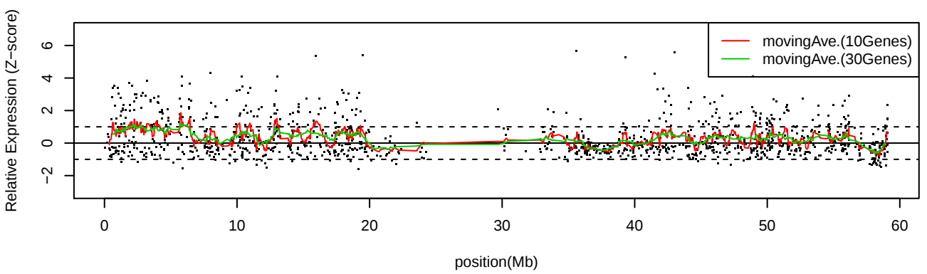
LC_C33 Chr19
