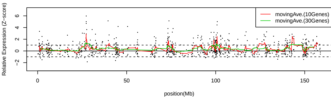
LC_C33 Chr7
