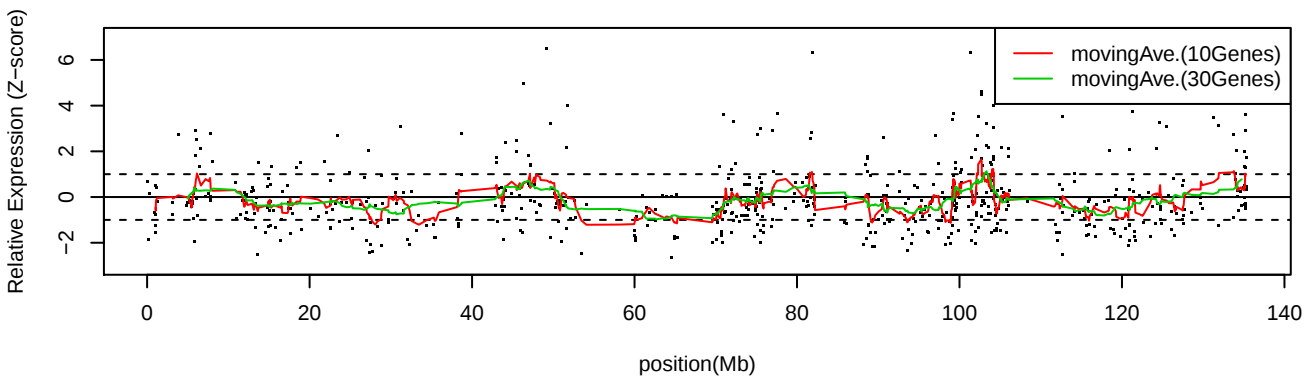
LC_S6 Chr10
