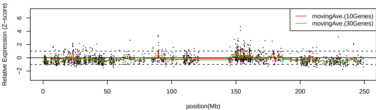
LC_C32 Chr1
