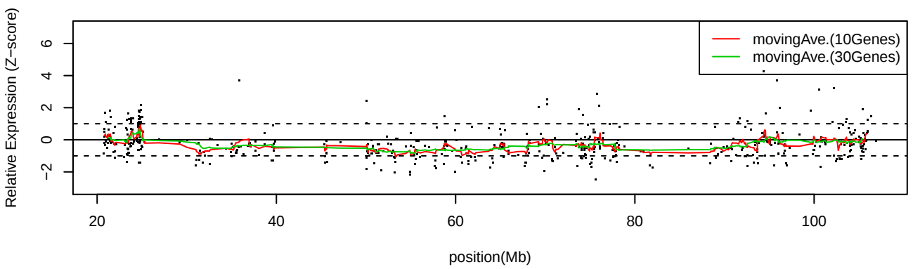
LC_S8 Chr14
