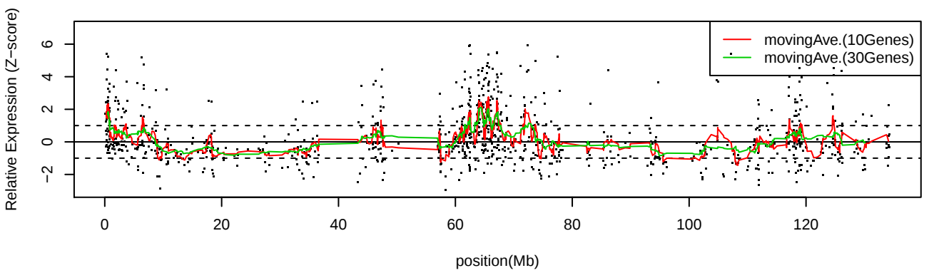
LC_S6 Chr11
