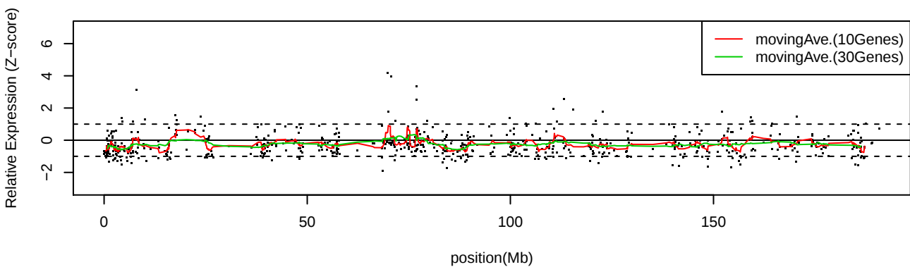
LC_C33 Chr4
