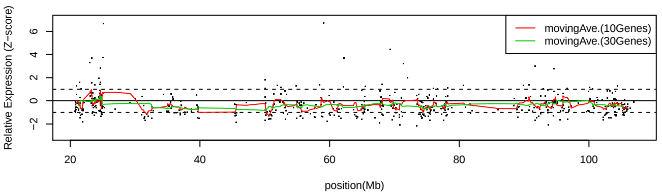
LC_S10 Chr14
