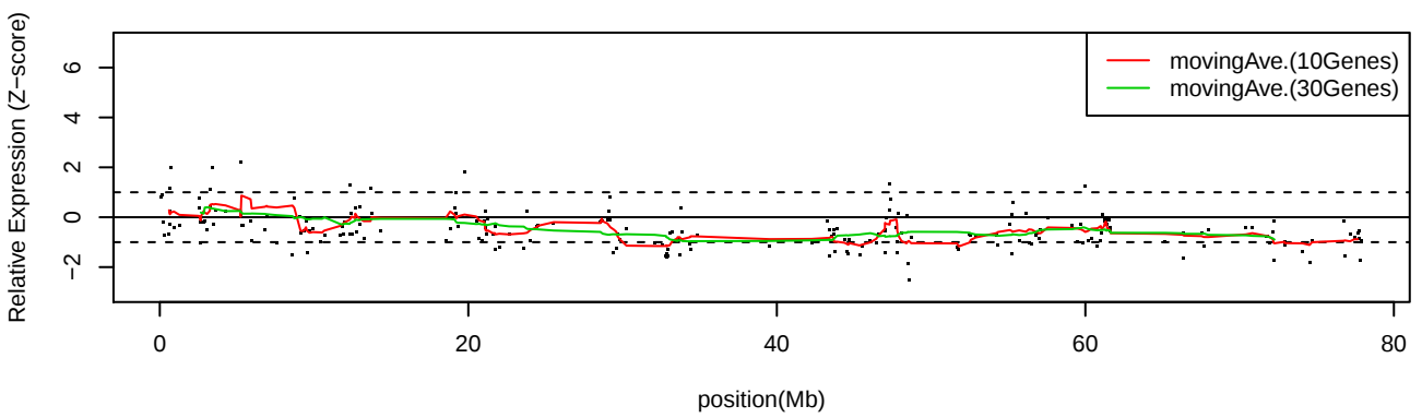
LC_C33 Chr18
