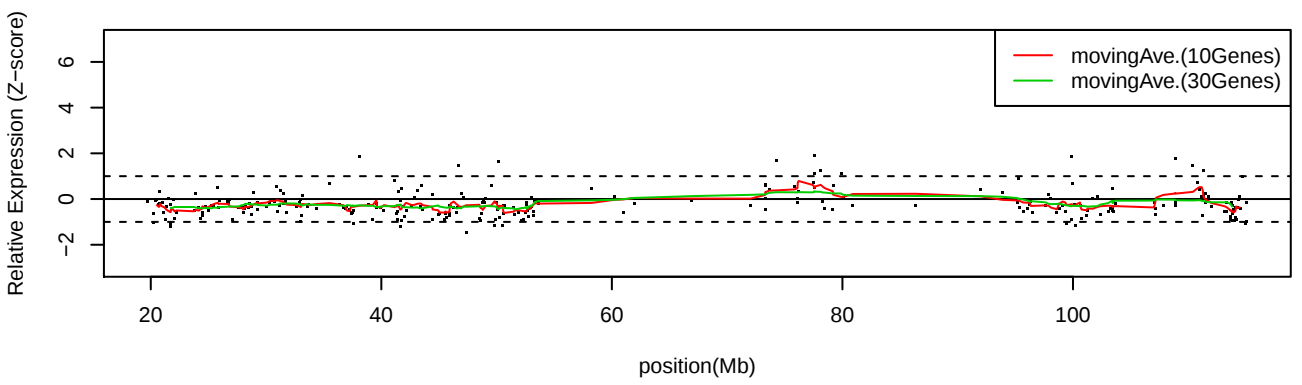
LC_C35 Chr13
