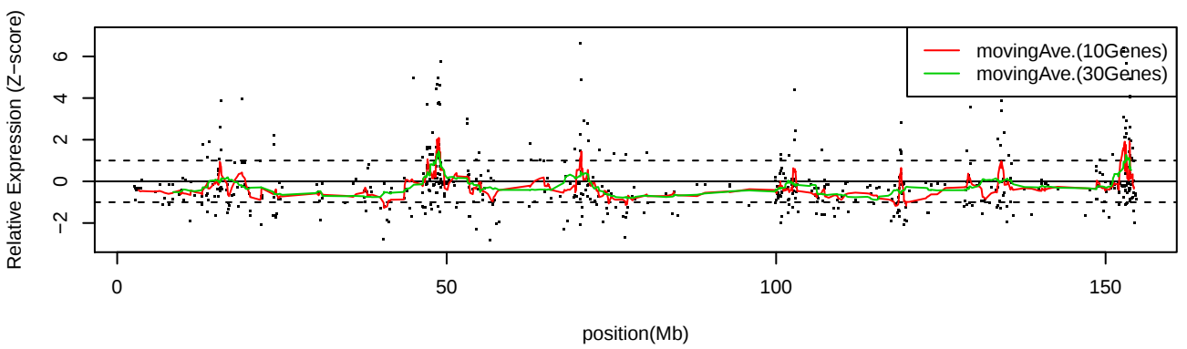
LC_S6 ChrX
