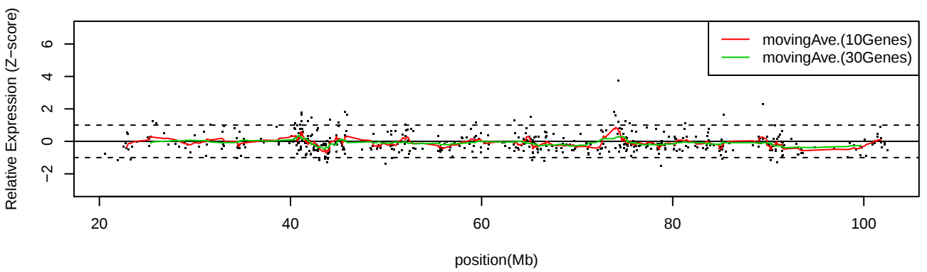
LC_C32 Chr15
