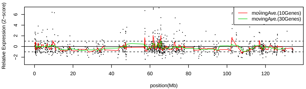
LC_S10 Chr11
