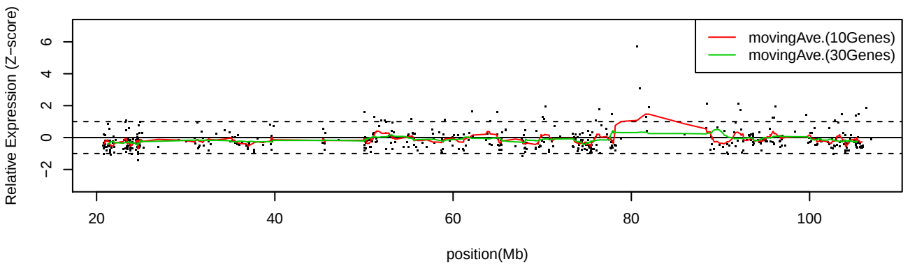
LC_C35 Chr14
