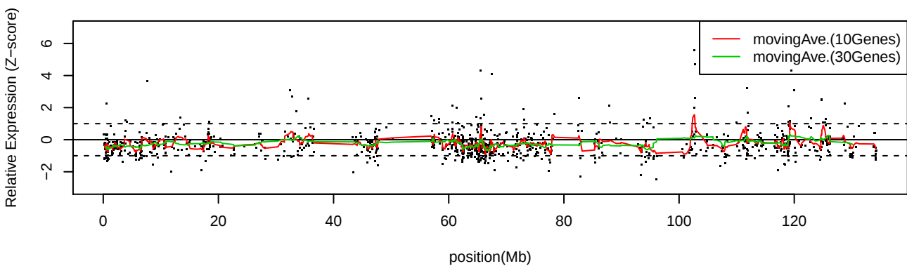
LC_C34 Chr11
