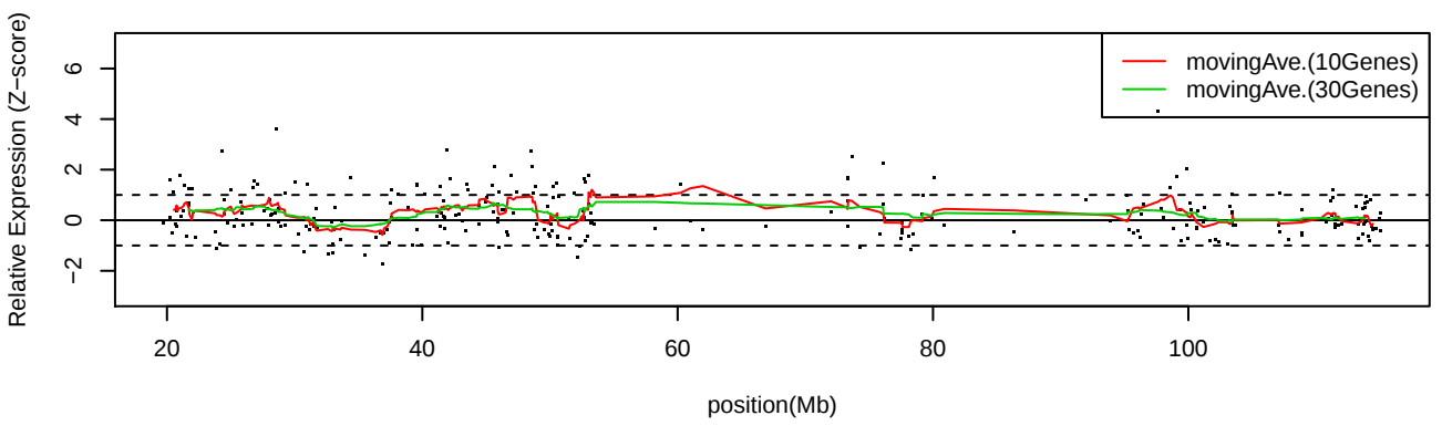
LC_C33 Chr13
