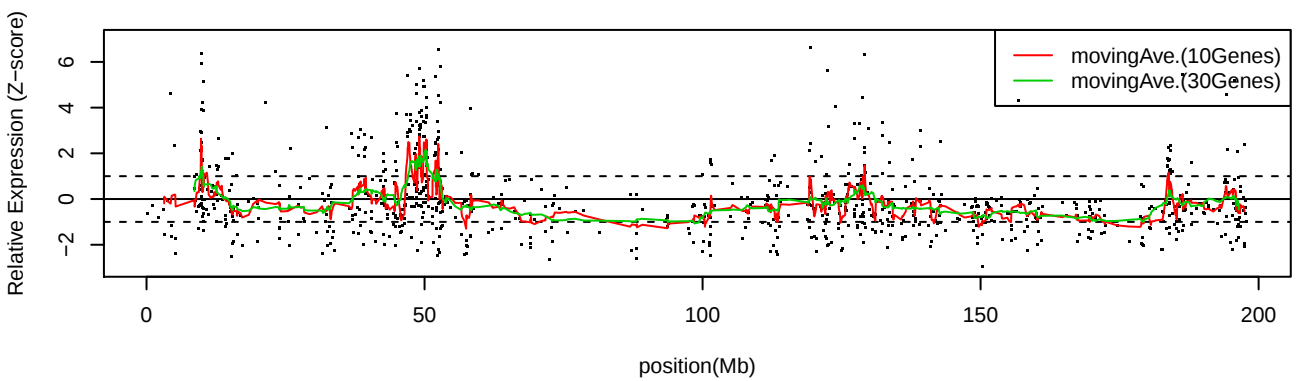
LC_S6 Chr3
