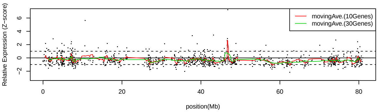
LC_C33 Chr17
