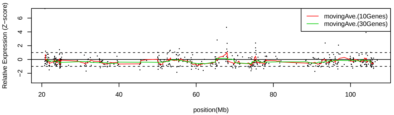
LC_C33 Chr14
