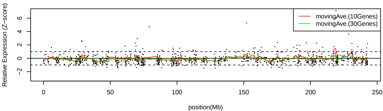
LC_C35 Chr2
