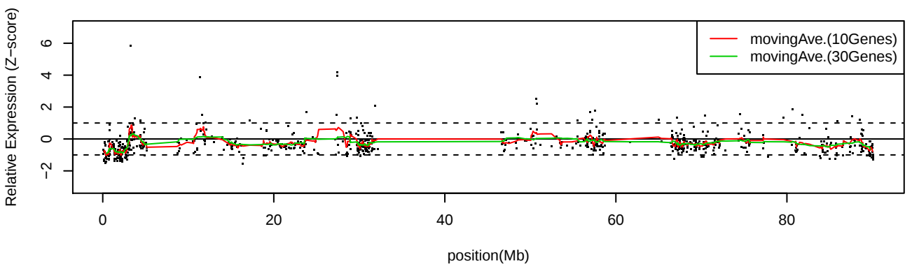
LC_C35 Chr16
