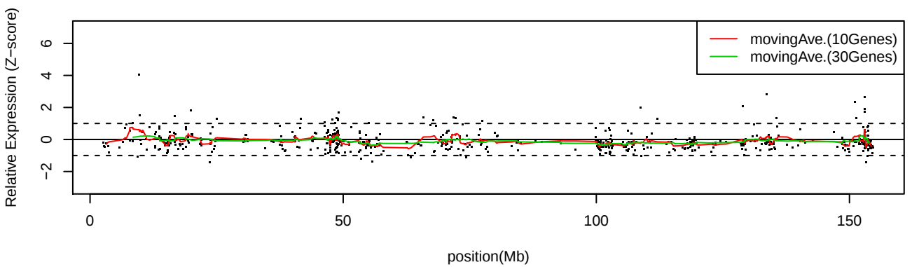
LC_C36 ChrX
