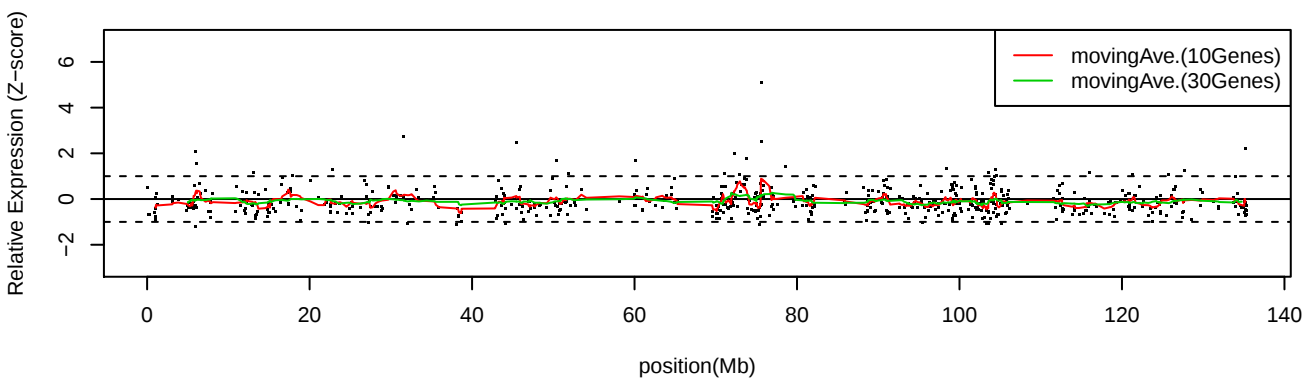
LC_C32 Chr10
