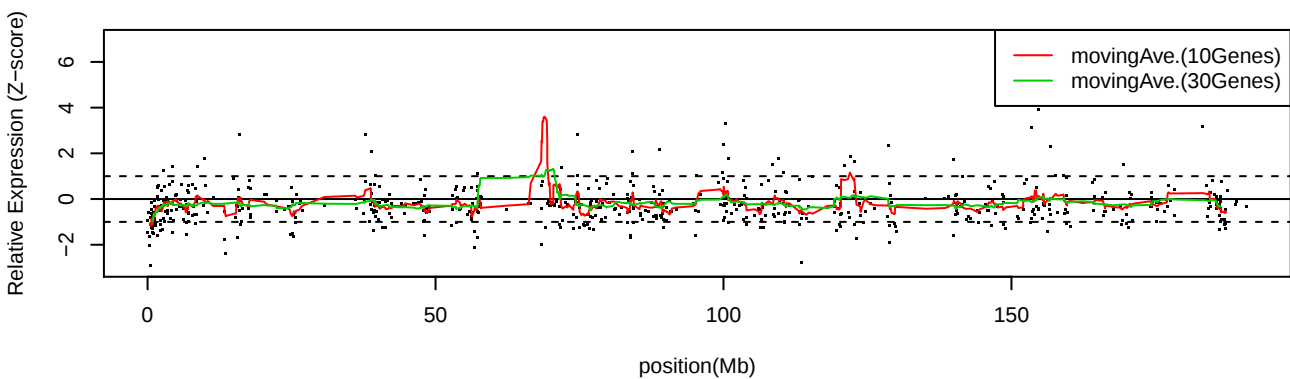
LC_C34 Chr4
