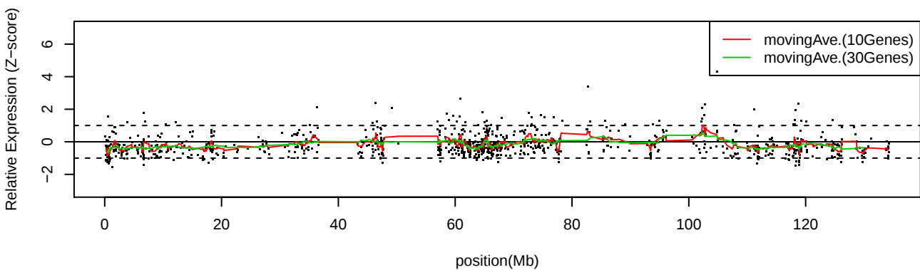
LC_C35 Chr11
