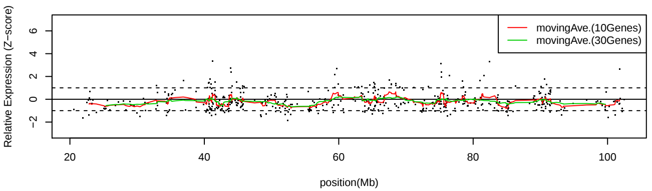
LC_C33 Chr15
