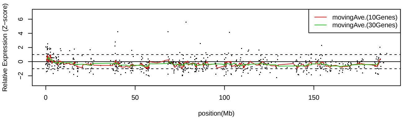
LC_S8 Chr4
