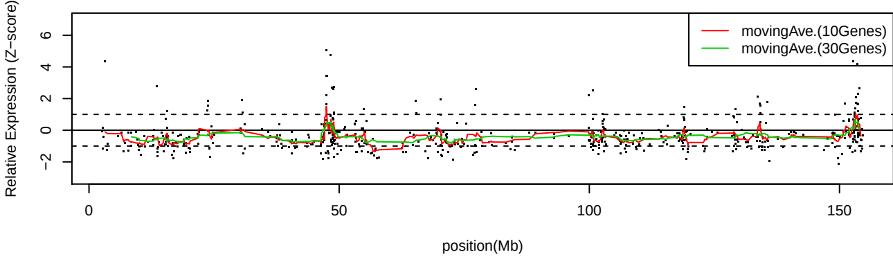
LC_S10 ChrX
