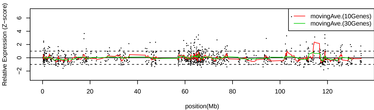
LC_C33 Chr11
