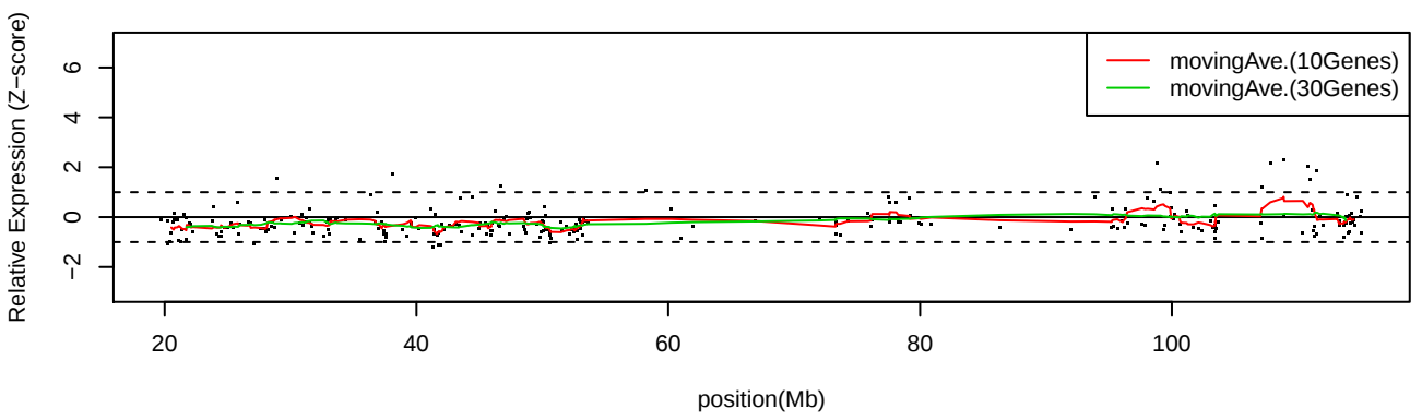
LC_C32 Chr13
