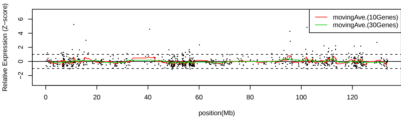
LC_C11 Chr12
