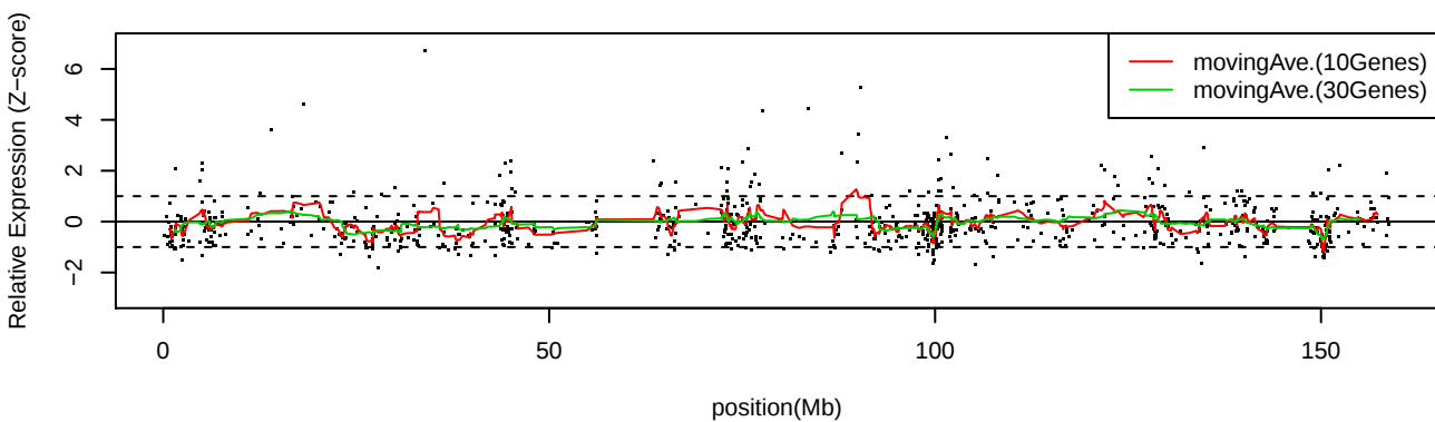
LC_C13 Chr7
