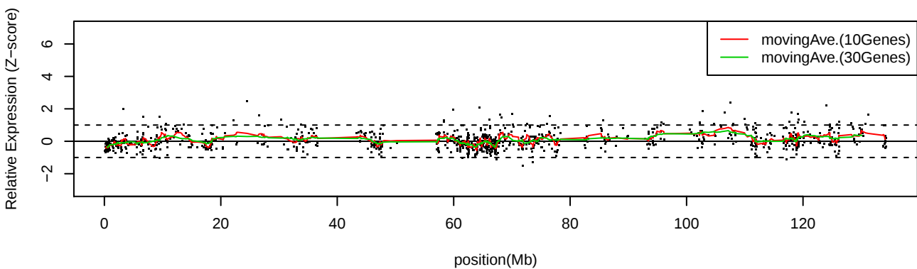
LC_C17 Chr11
