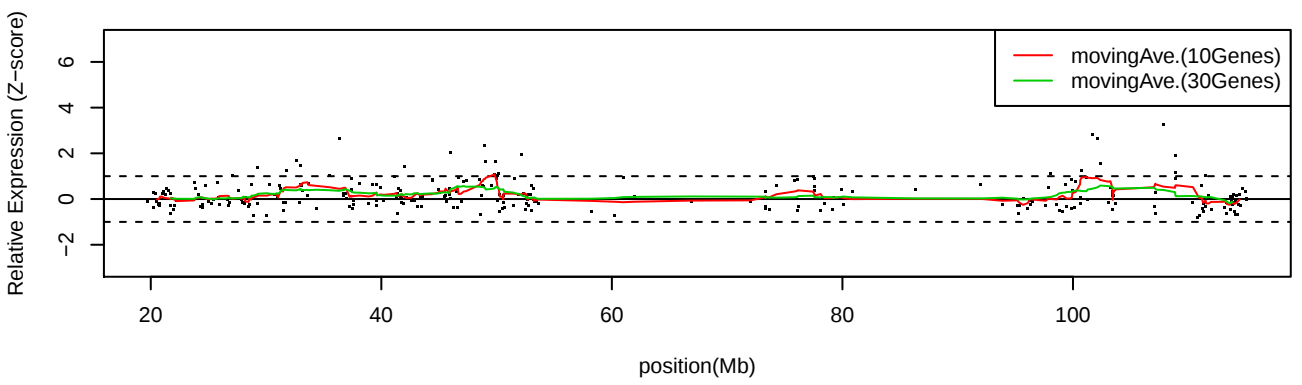
LC_C12 Chr13
