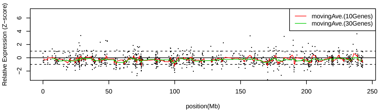
LC_C20 Chr2
