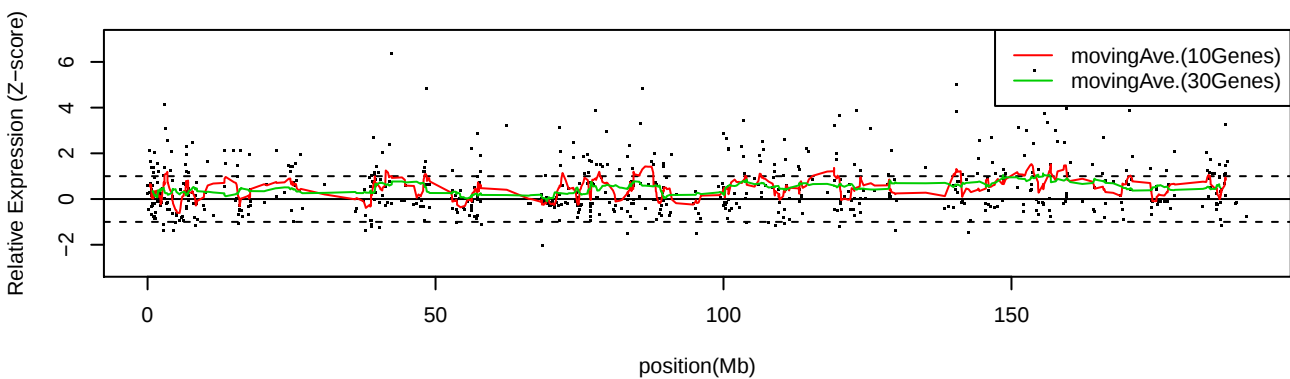
LC_C15 Chr4
