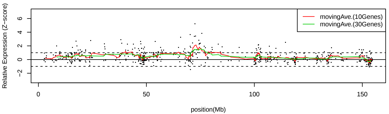
LC_C16 ChrX
