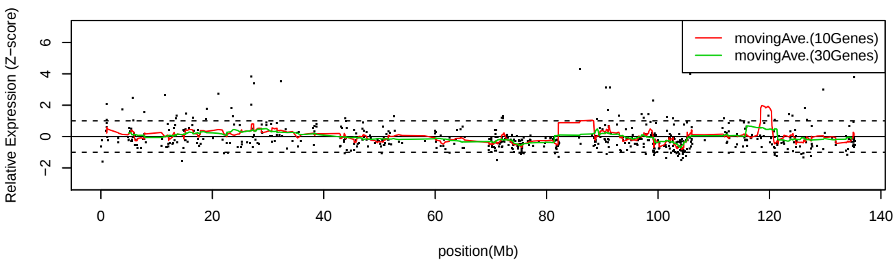
LC_C19 Chr10
