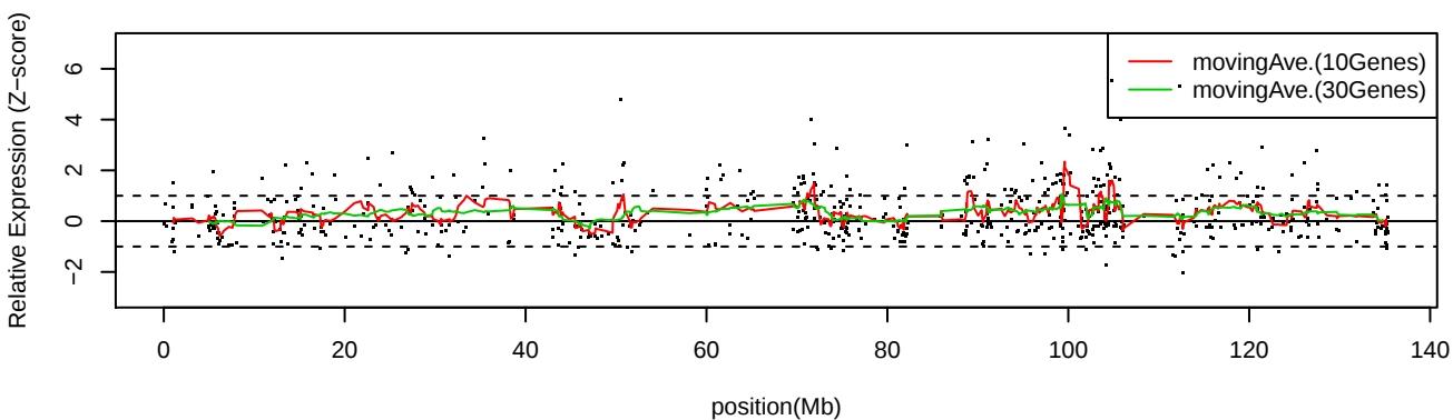
LC_C13 Chr10
