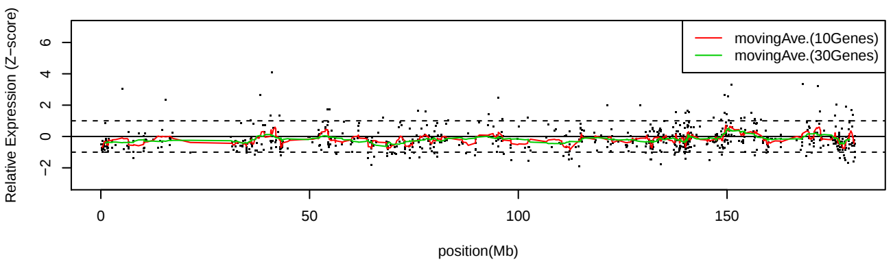
LC_C20 Chr5
