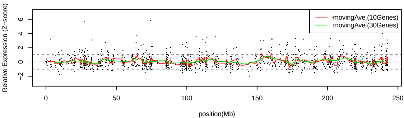
LC_C15 Chr2
