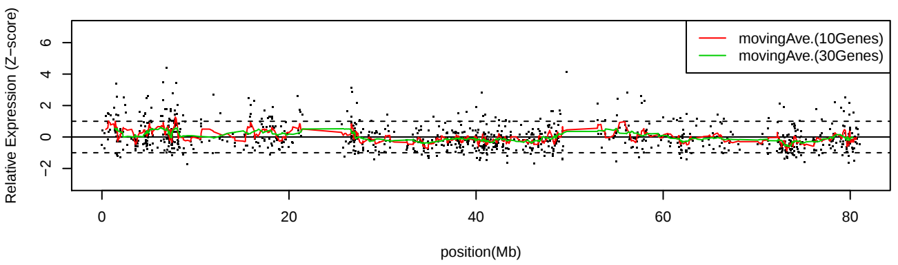
LC_C15 Chr17
