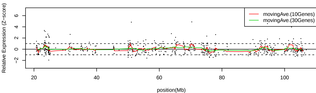
LC_C13 Chr14
