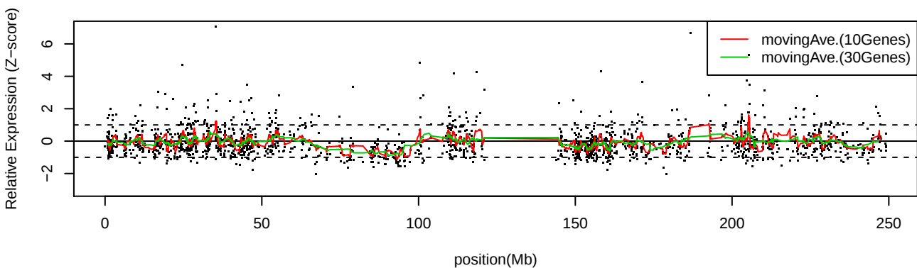
LC_C13 Chr1
