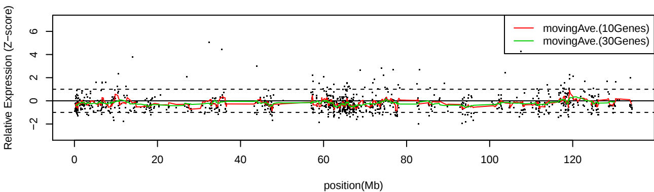
LC_C20 Chr11
