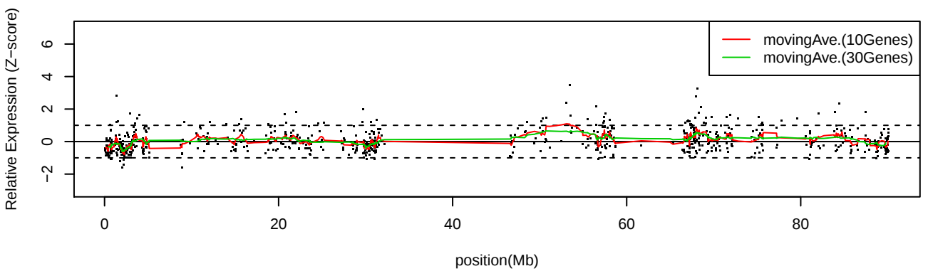
LC_C16 Chr16
