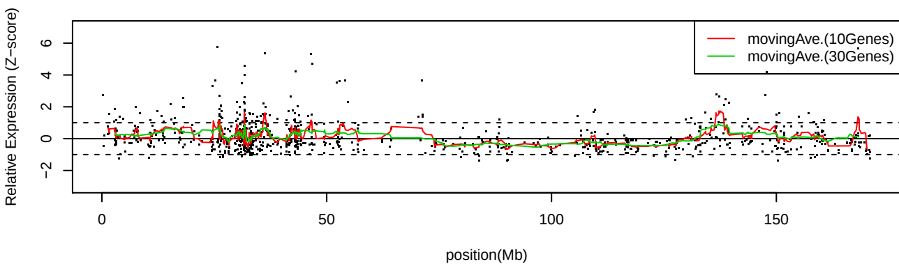
LC_C19 Chr6
