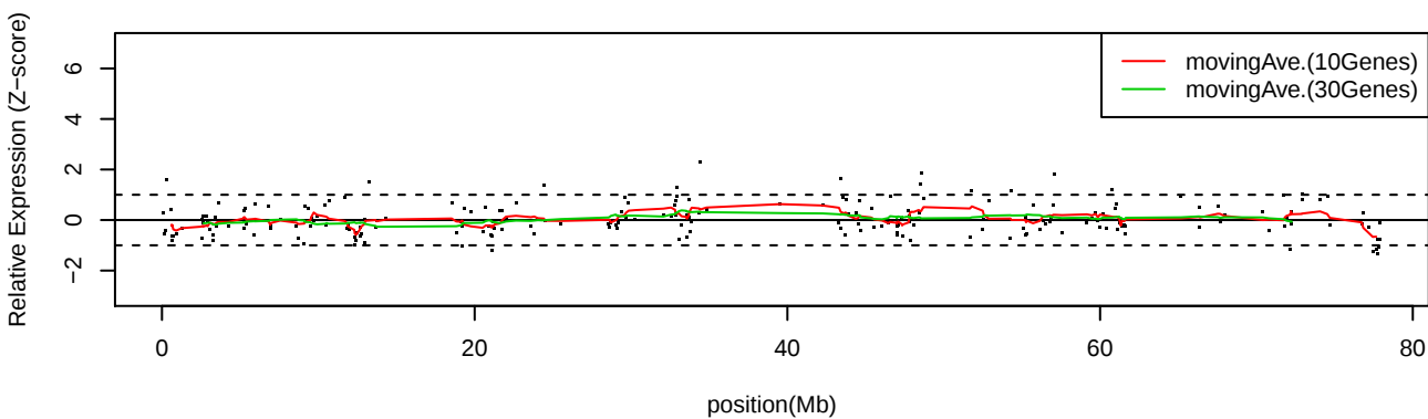
LC_C16 Chr18
