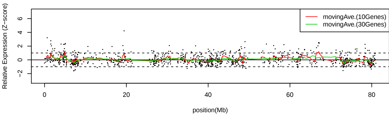
LC_C16 Chr17
