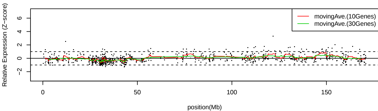
LC_C17 Chr6
