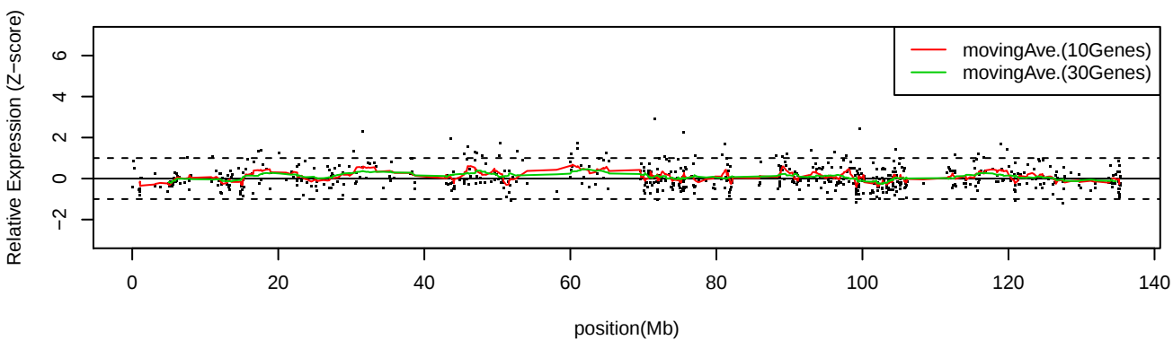
LC_C17 Chr10
