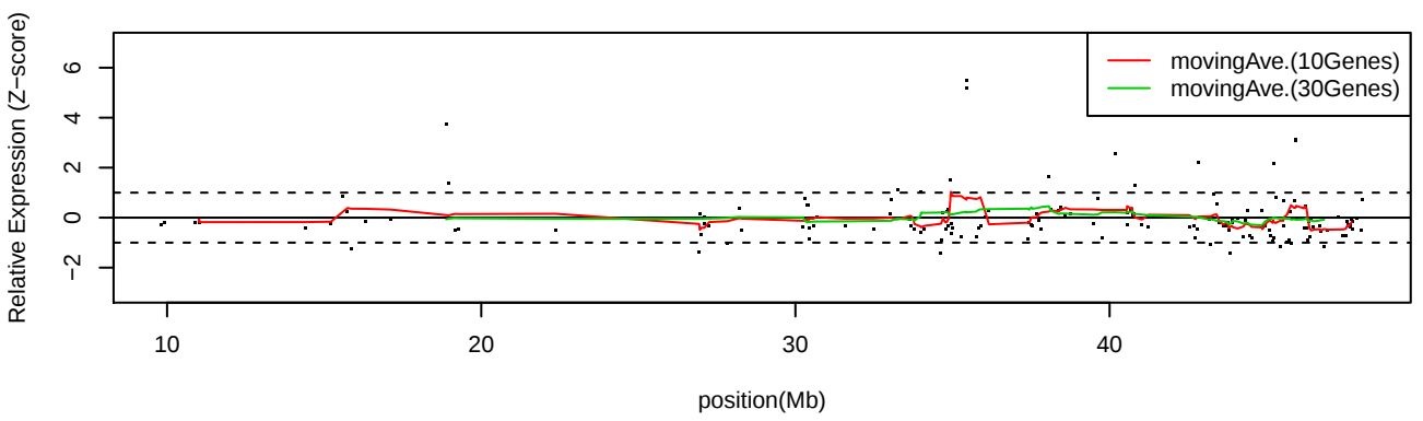
LC_C15 Chr21
