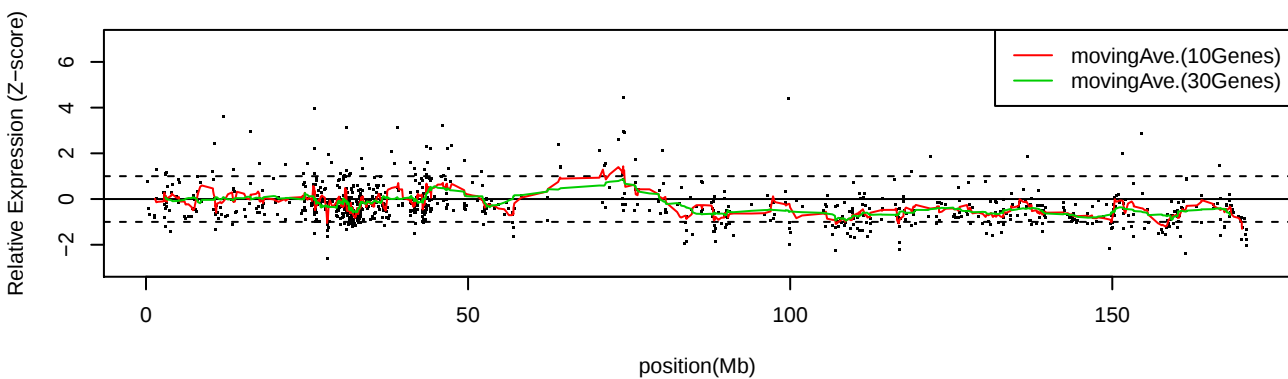
LC_C13 Chr6
