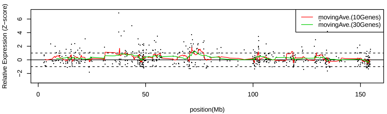
LC_C15 ChrX
