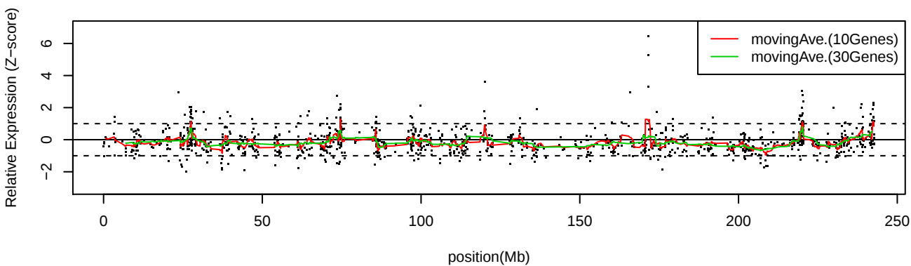
LC_C14 Chr2
