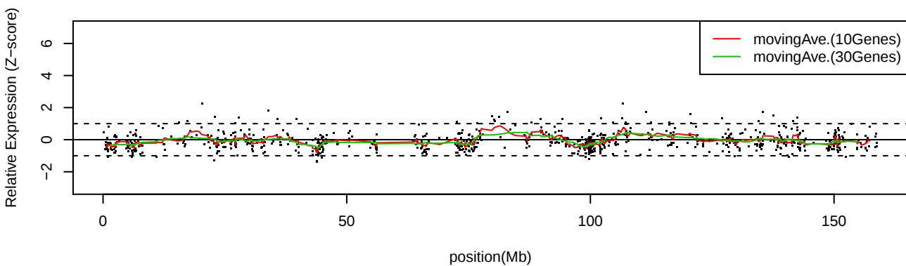
LC_C17 Chr7
