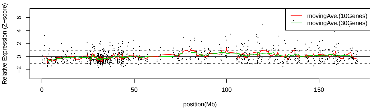
LC_C15 Chr6
