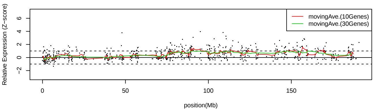
LC_C12 Chr4
