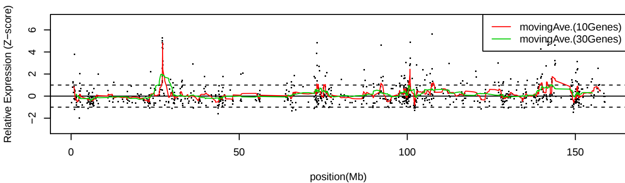
LC_C19 Chr7
