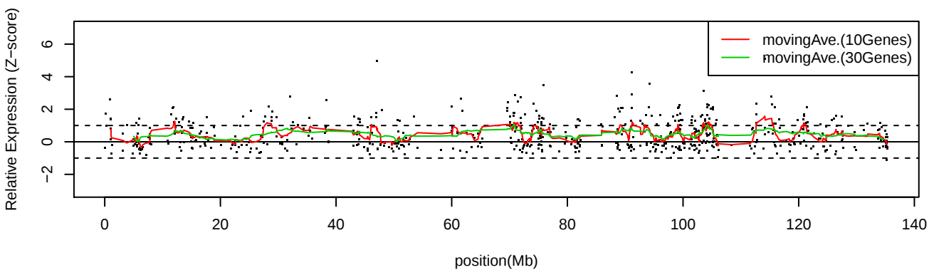
LC_C11 Chr10
