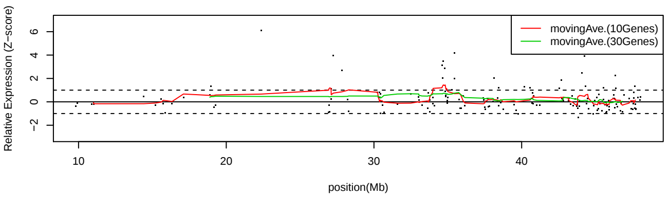
LC_C13 Chr21
