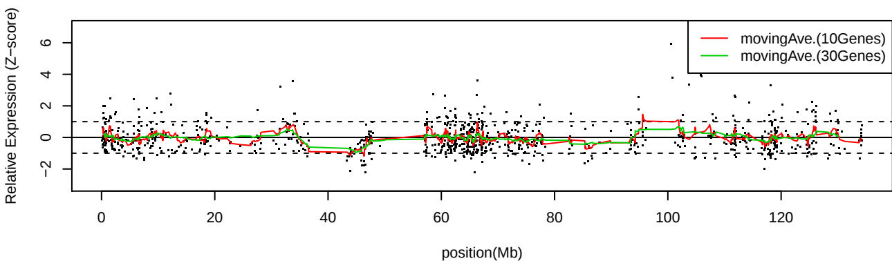
LC_C13 Chr11
