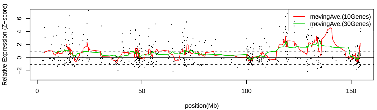
LC_C18 ChrX
