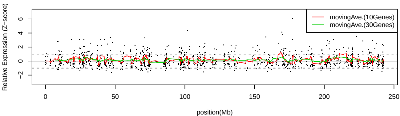
LC_C13 Chr2
