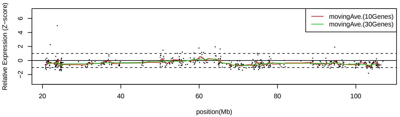
LC_C11 Chr14
