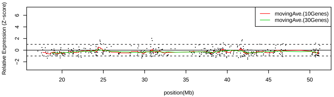
LC_C16 Chr22
