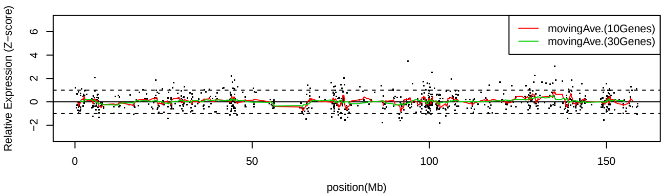
LC_C20 Chr7
