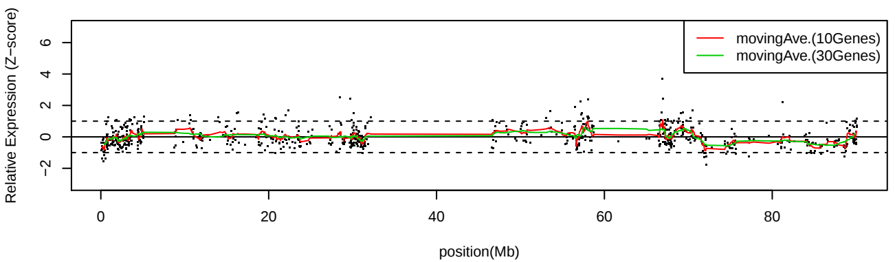
LC_C11 Chr16
