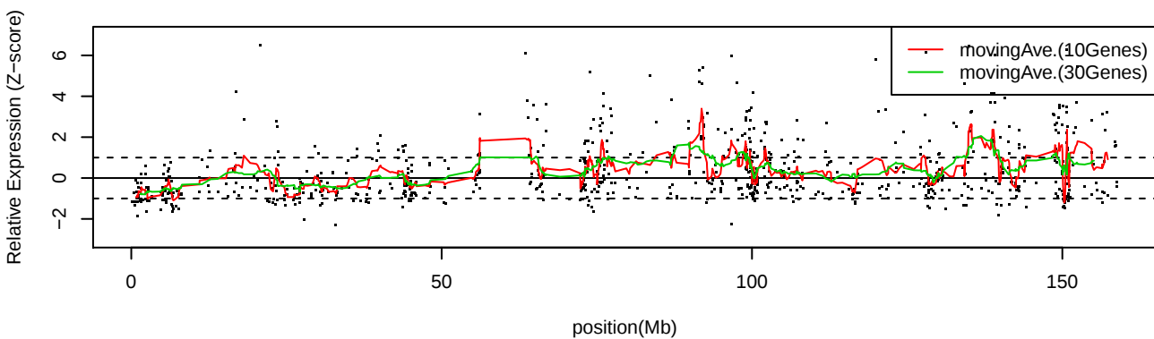
LC_C18 Chr7
