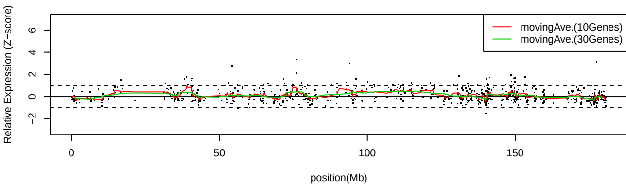
LC_C17 Chr5
