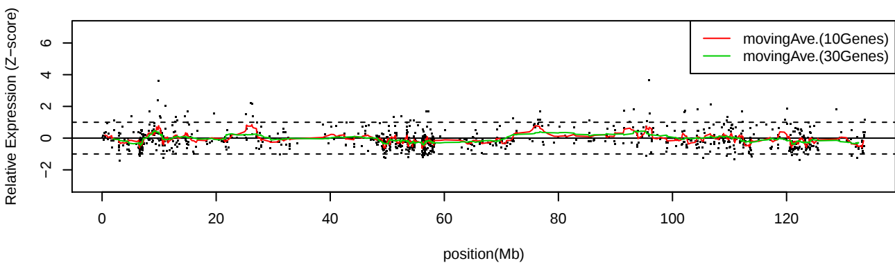
LC_C16 Chr12
