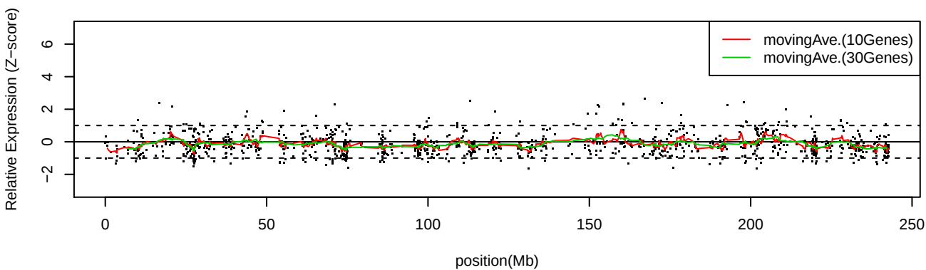
LC_C16 Chr2
