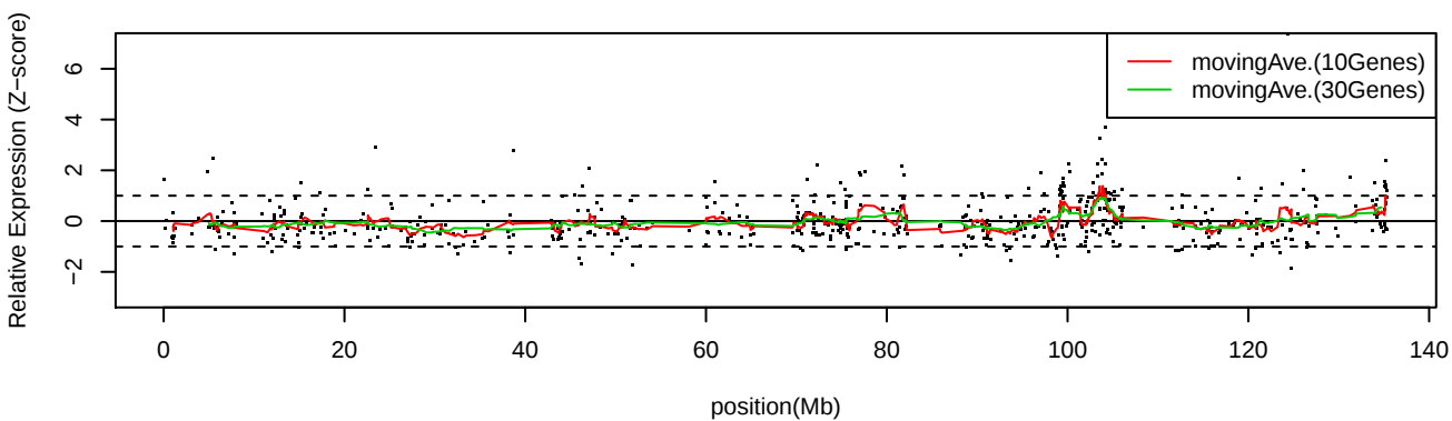
LC_C14 Chr10
