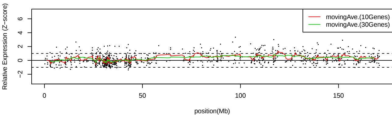
LC_C16 Chr6
