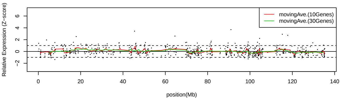
LC_C16 Chr10
