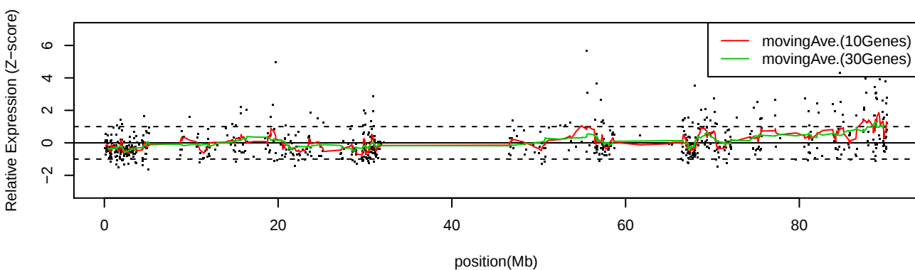
LC_C13 Chr16
