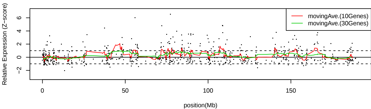
LC_C13 Chr4
