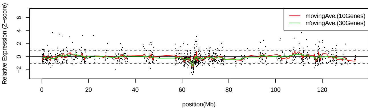
LC_C15 Chr11
