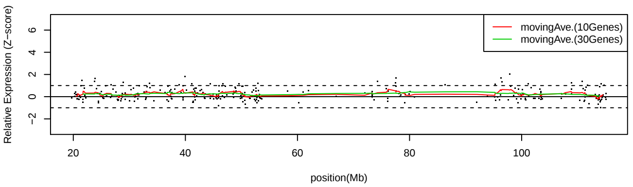
LC_C17 Chr13
