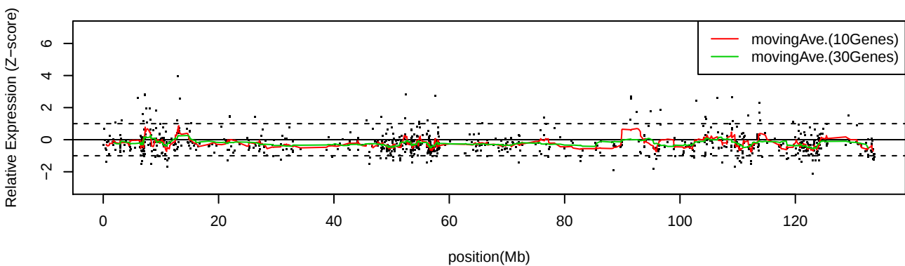
LC_C20 Chr12
