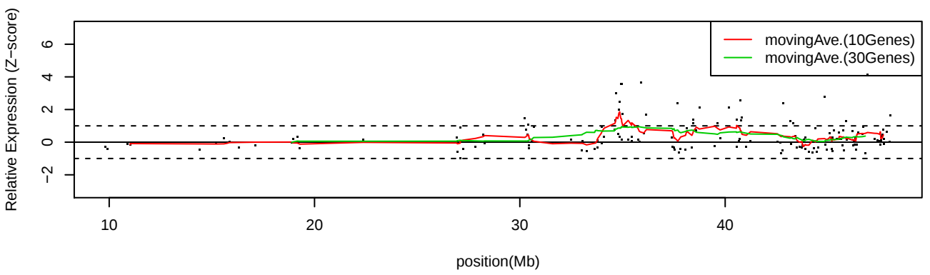
LC_C16 Chr21
