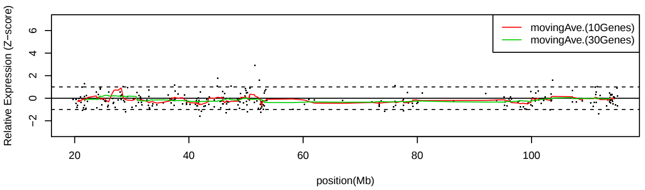
LC_C14 Chr13
