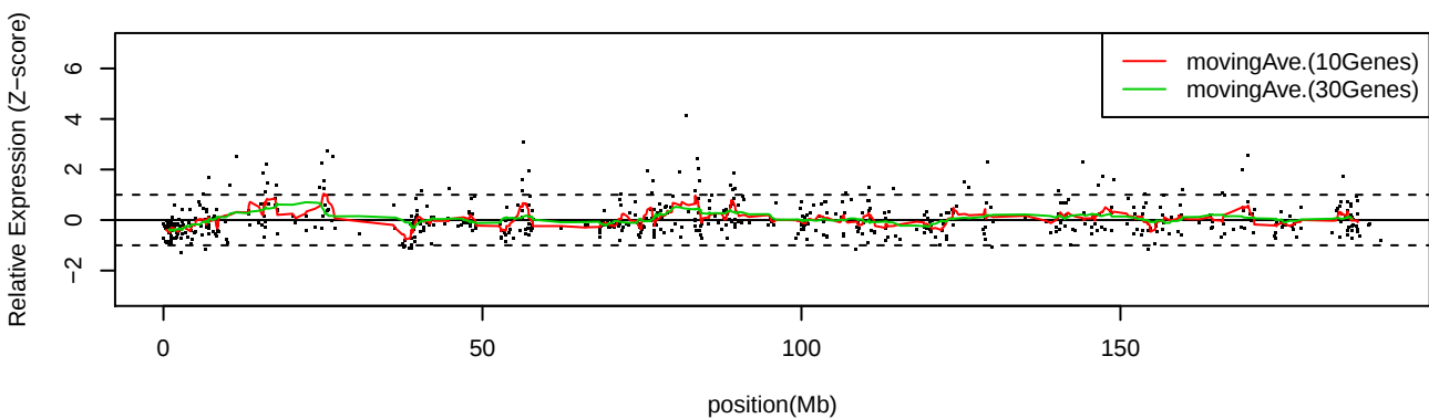
LC_C11 Chr4
