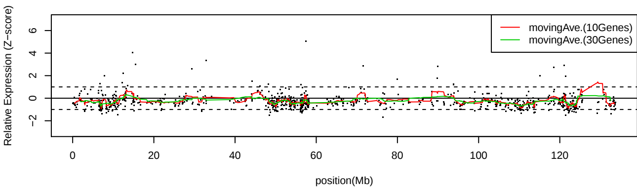
LC_C19 Chr12
