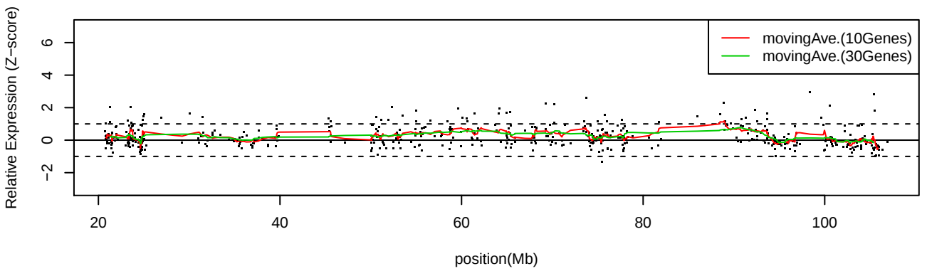
LC_C12 Chr14
