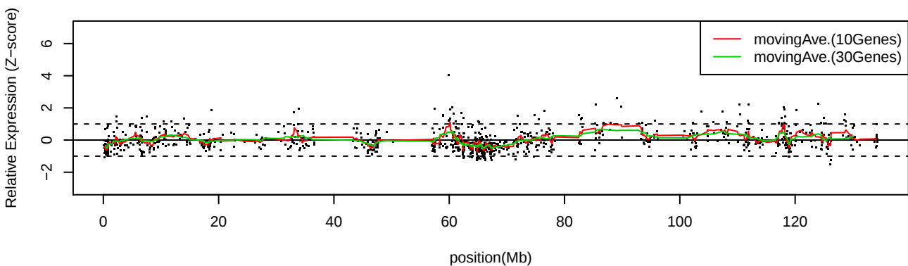
LC_C12 Chr11
