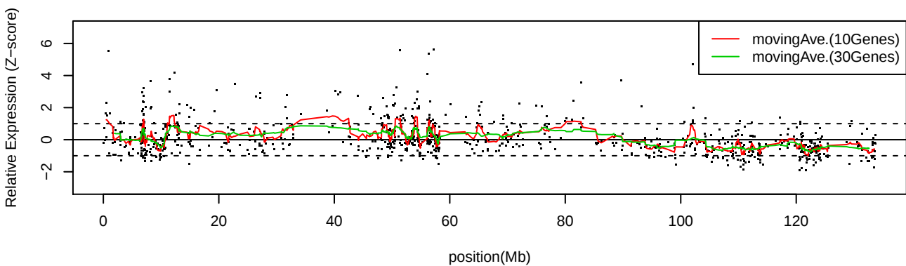
LC_C15 Chr12
