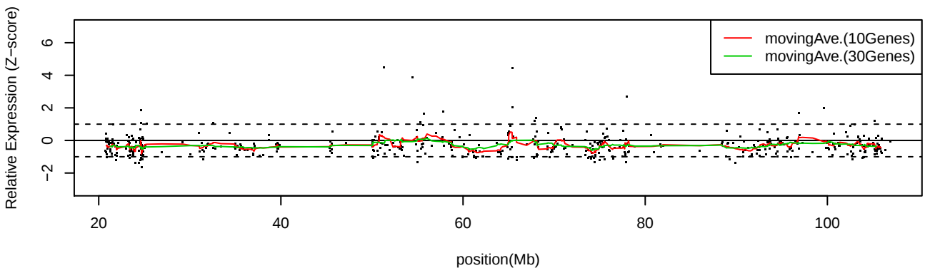
LC_C19 Chr14
