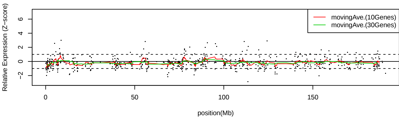
LC_C20 Chr4
