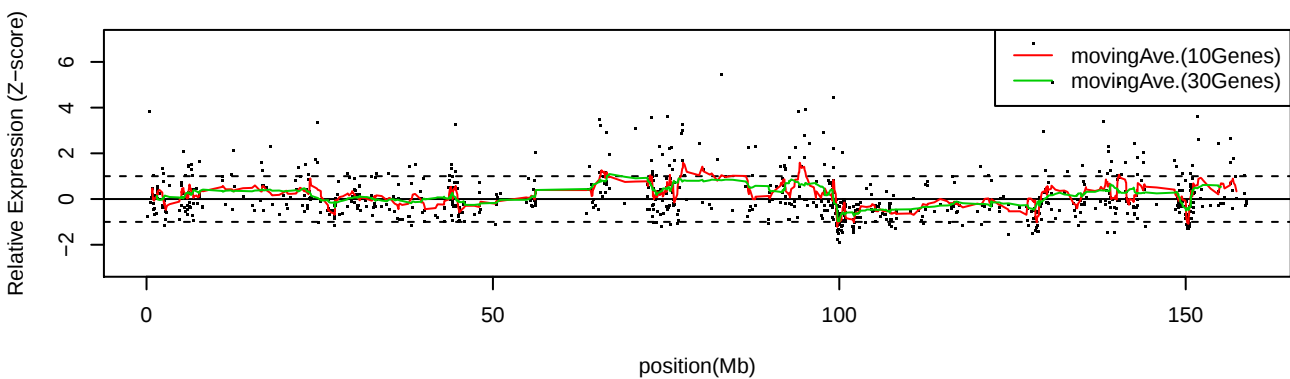
LC_C15 Chr7
