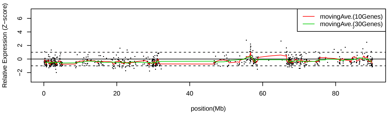
LC_C20 Chr16
