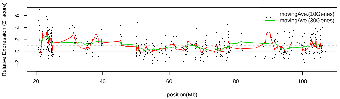
LC_C18 Chr14
