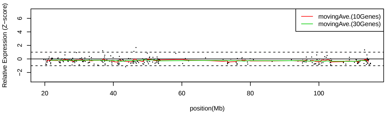
LC_C11 Chr13
