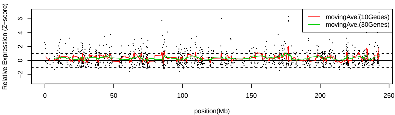
LC_C19 Chr2
