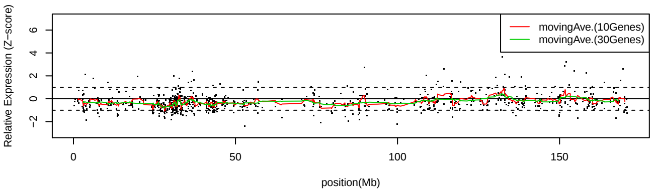
LC_C20 Chr6
