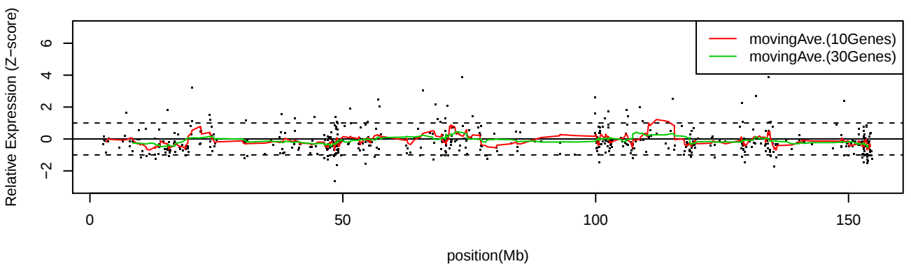
LC_C13 ChrX
