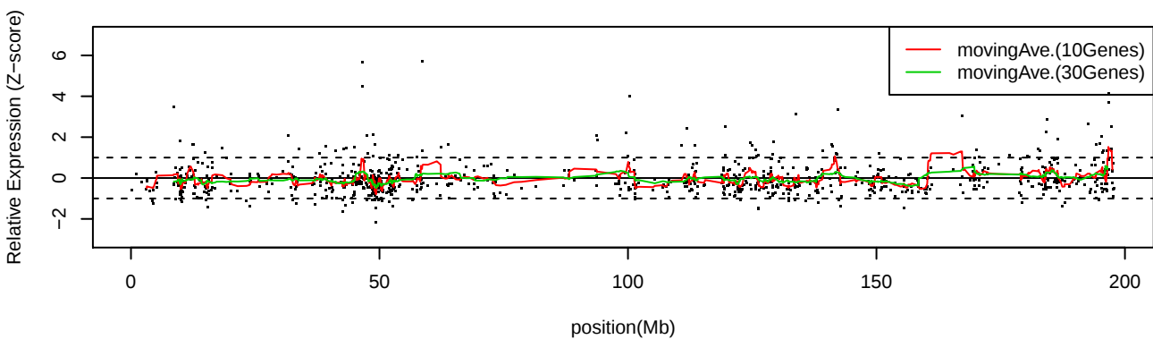
LC_C19 Chr3
