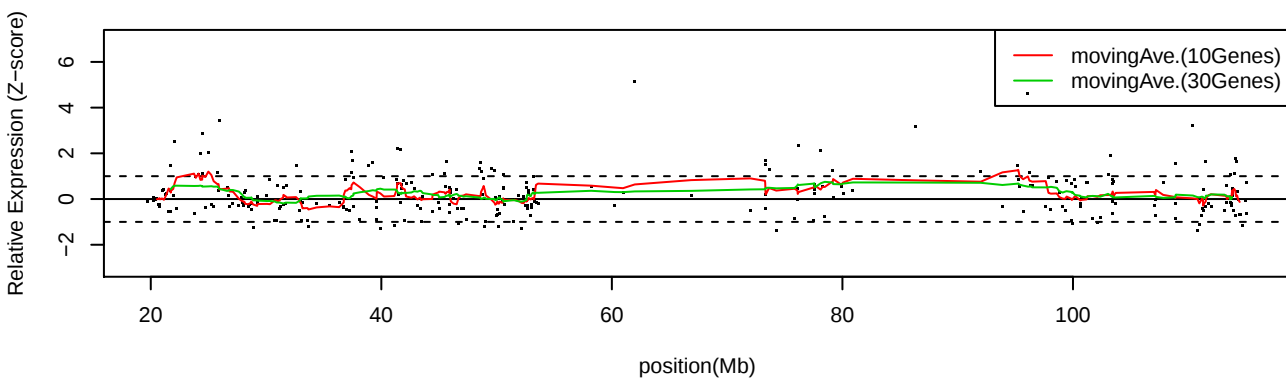
LC_C13 Chr13
