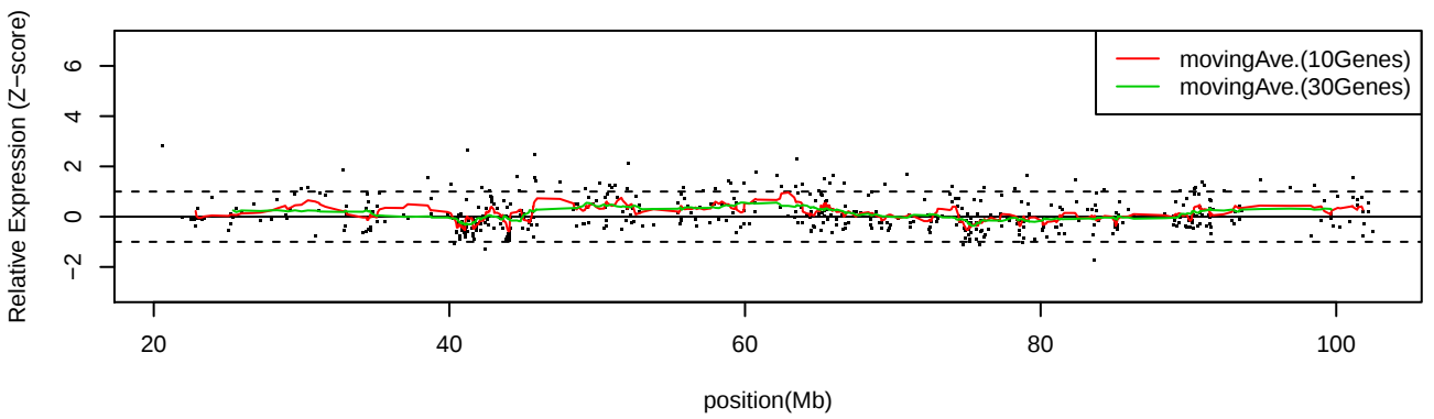
LC_C17 Chr15
