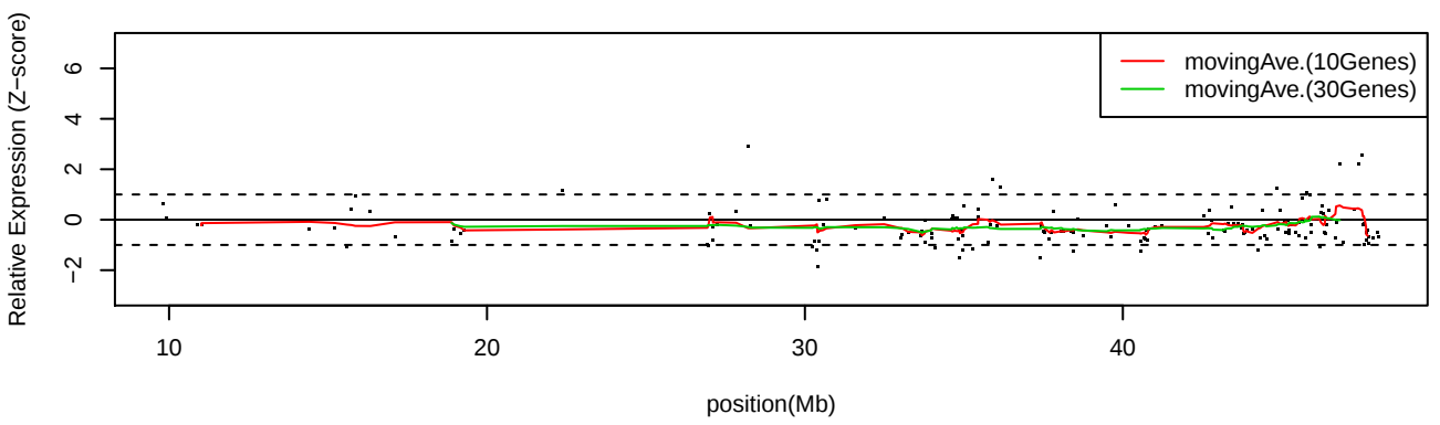
LC_C20 Chr21
