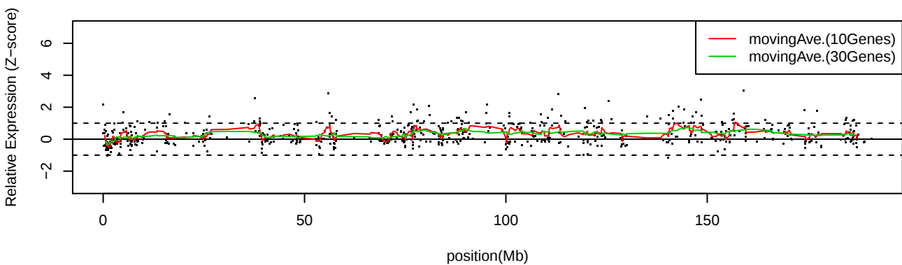
LC_C17 Chr4
