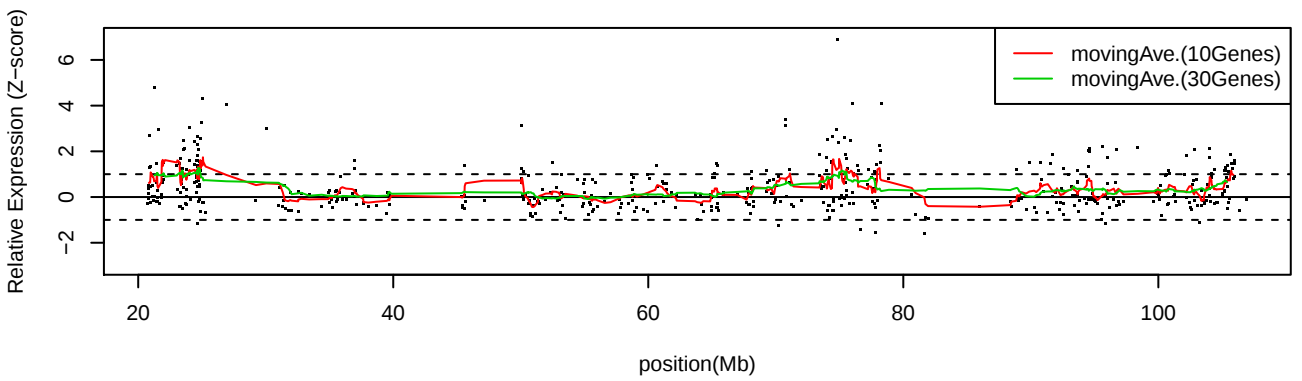
LC_C14 Chr14
