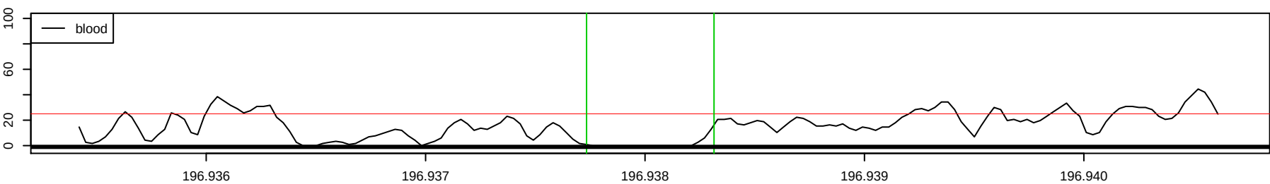
Chr 3 : 196937734 – 196938314 , 581 bp
