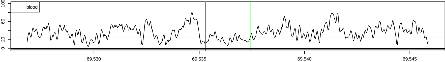
Chr 16 : 69535301 – 69537421 , 2121 bp
