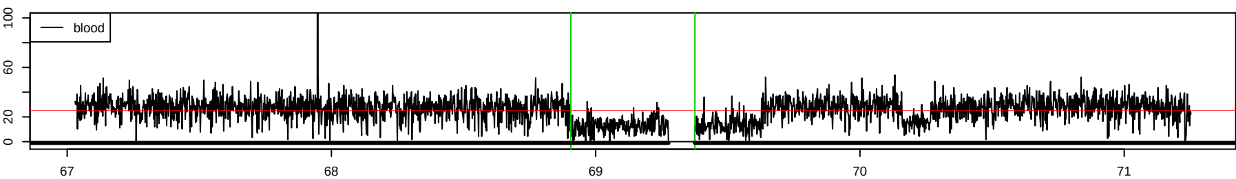
Chr 4 : 68906080 – 69375493 , 469414 bp
