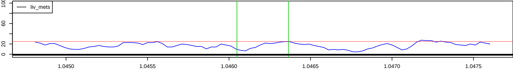
Chr 10 : 1046049 – 1046364 , 316 bp
