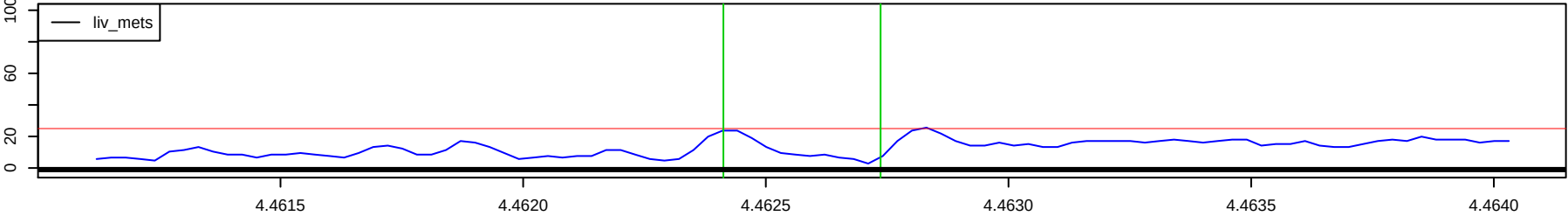
Chr 19 : 4462413 – 4462736 , 324 bp
