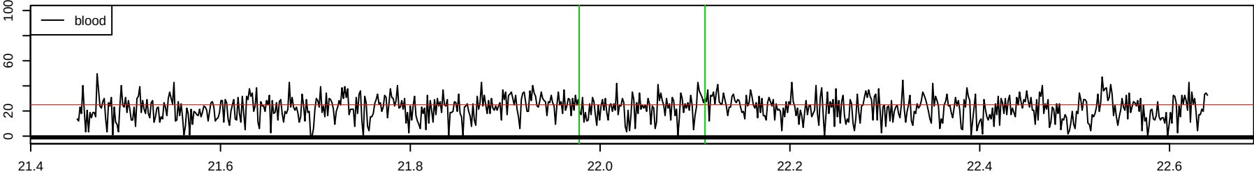
Chr 19 : 21977934 – 22110543 , 132610 bp
