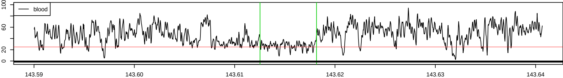
Chr 1 : 143612529 – 143618160 , 5632 bp
