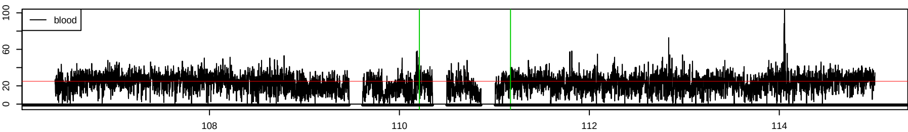
Chr 2 : 110210032 – 111169571 , 959540 bp
