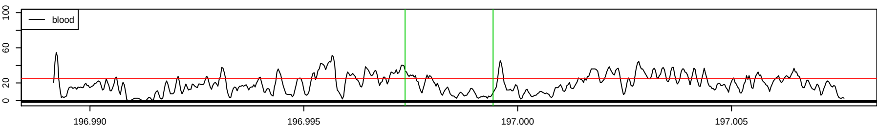
Chr 3 : 196997367 – 196999424 , 2058 bp
