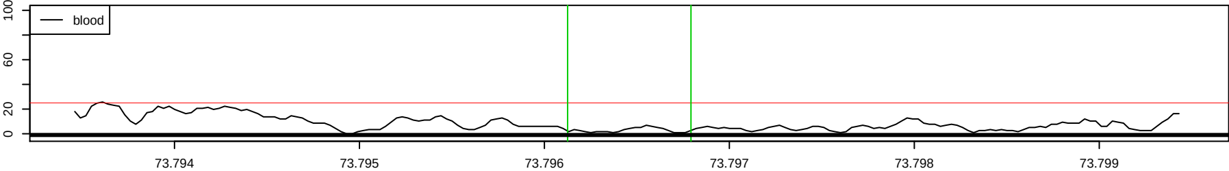
Chr 16 : 73796126 – 73796792 , 667 bp
