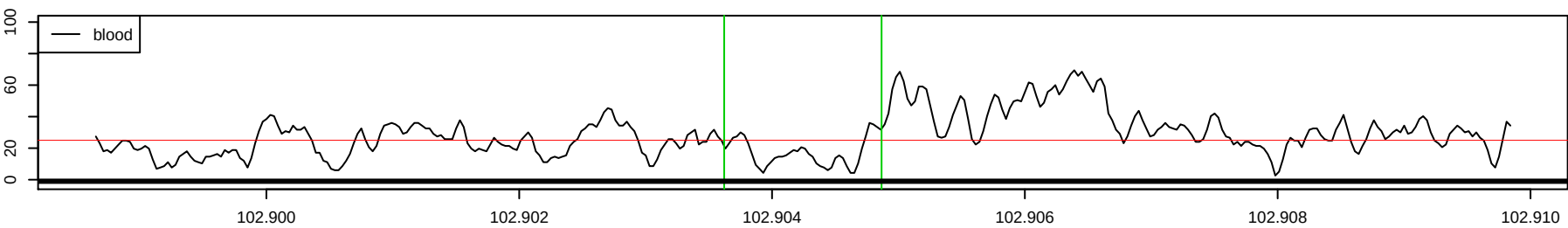
Chr 12 : 102903622 – 102904866 , 1245 bp
