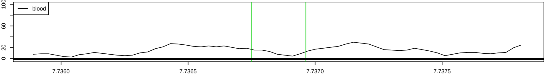
Chr 19 : 7736749 – 7736963 , 215 bp
