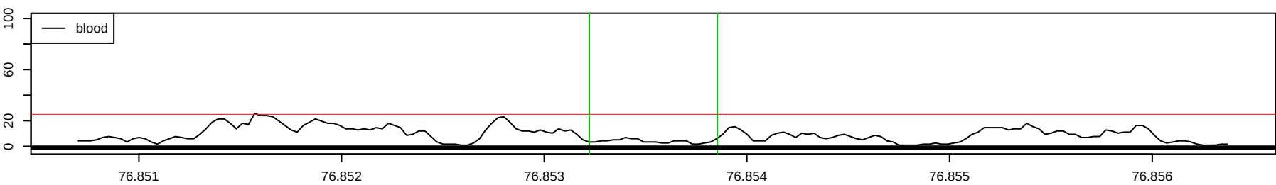
Chr 15 : 76853223 – 76853854 , 632 bp
