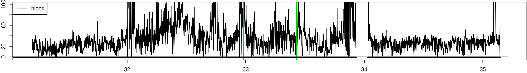
Chr 16 : 32980051 – 33426267 , 446217 bp
