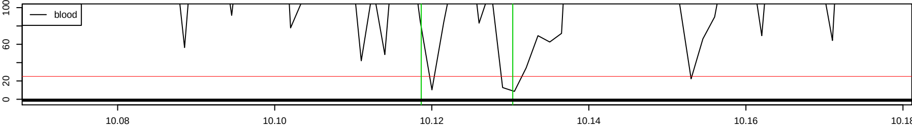
Chr 21 : 10118656 – 10130310 , 11655 bp
