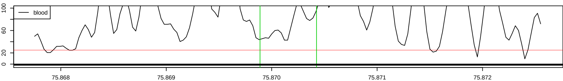
Chr 3 : 75869890 – 75870425 , 536 bp
