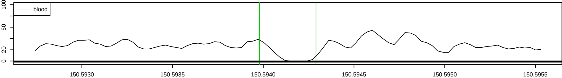
Chr 1 : 150593980 – 150594290 , 311 bp
