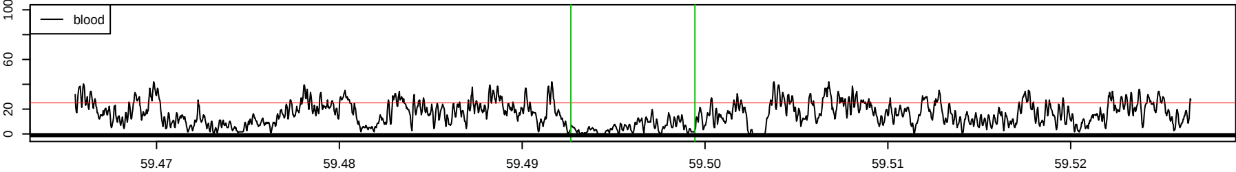
Chr 19 : 59492662 – 59499446 , 6785 bp
