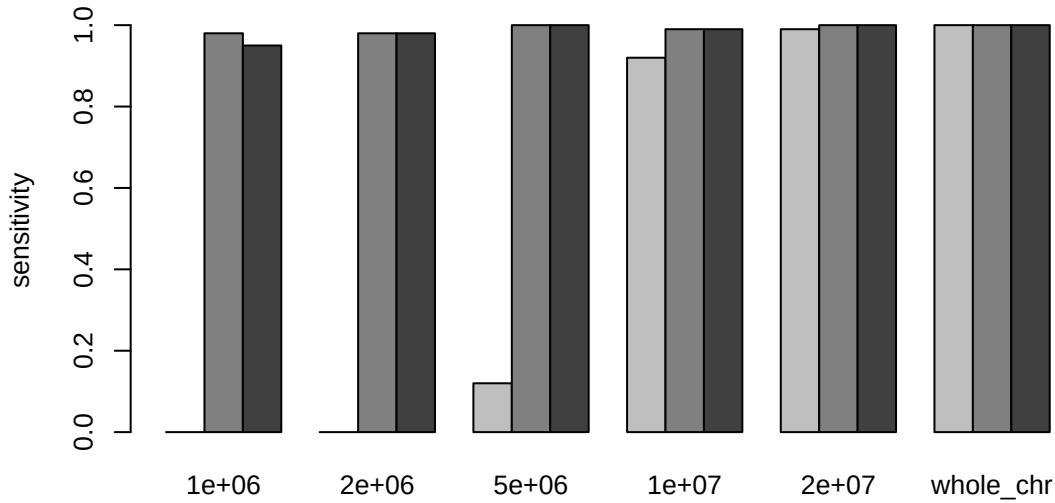
Isodisomy from SNP
