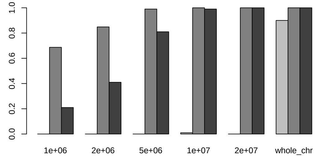
Isodisomy from exome
