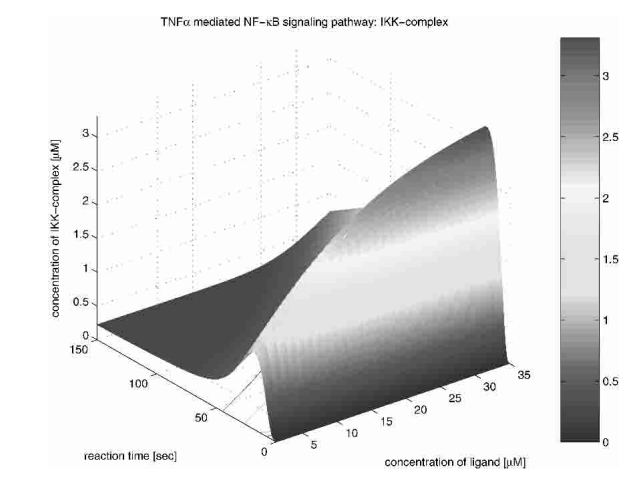
Figure 22 IKK complex.
